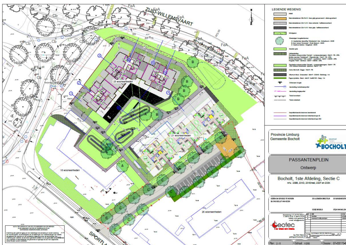
Figuur 2: Plan van de geplande werken (Q-Bus Architectenbureau, 2021)
