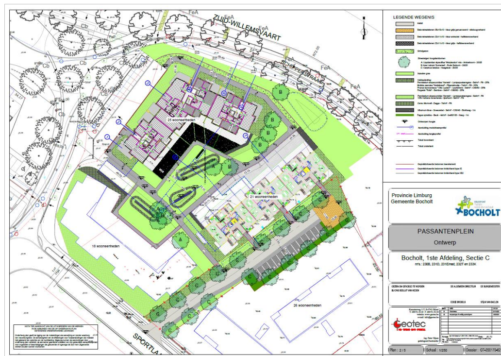
Figuur 5: Inplantingsplan van de geplande werken (opdrachtgever, 2021)
