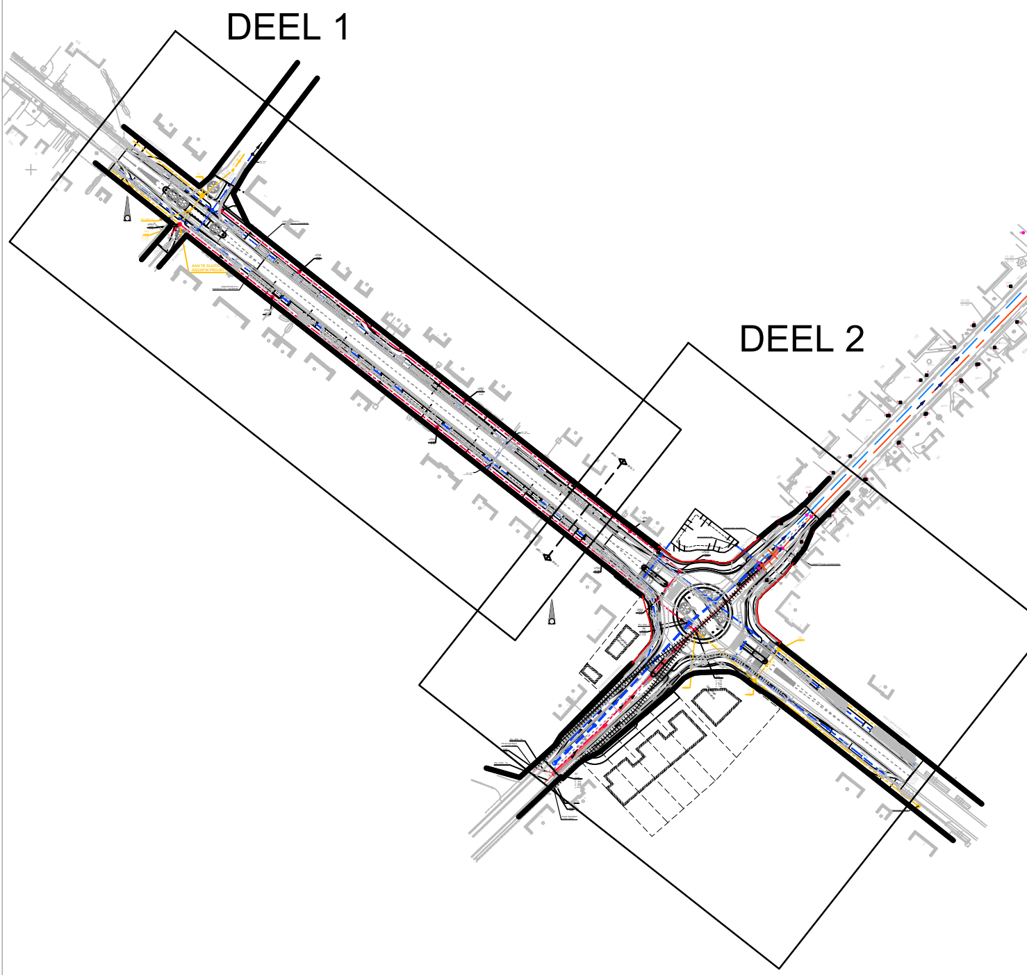
OVERZICHTSPLAN schaal : 1 / 2500
