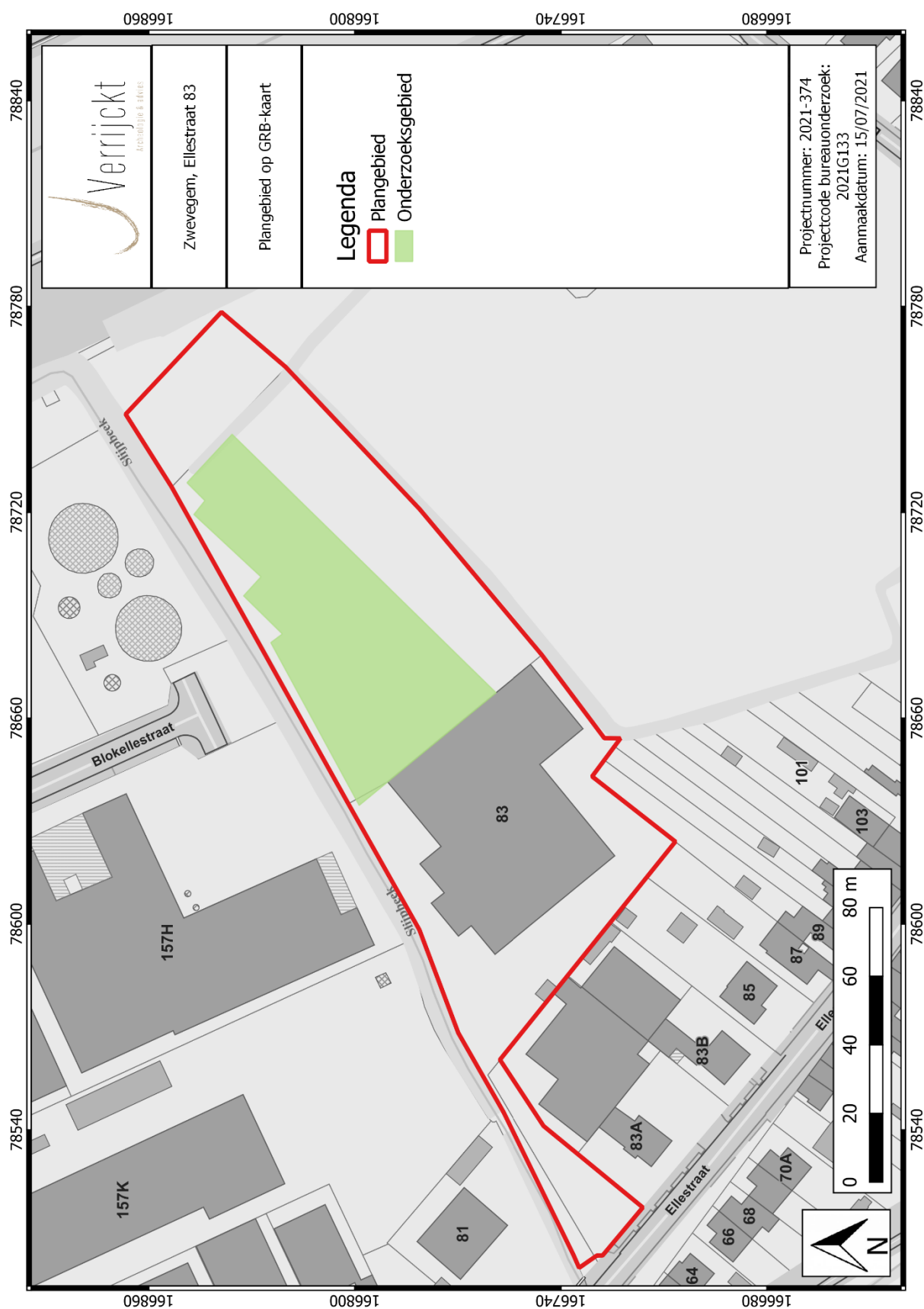
Figuur 3: Plangebied met weergave onderzoeksgebied
