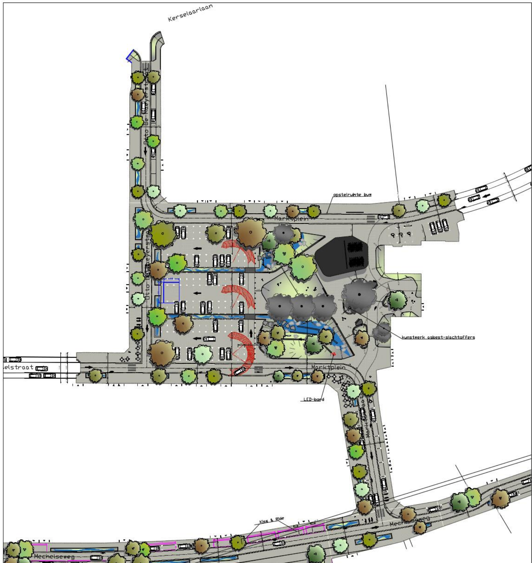
Figuur 4: Ontwerpplan van het Marktplein
