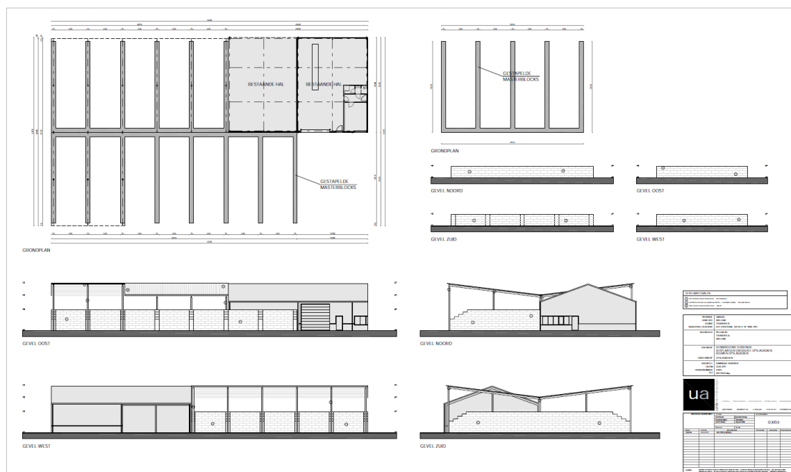
Figuur 3: Bouwplannen van de opslagboxen (opdrachtgever, 2021)
