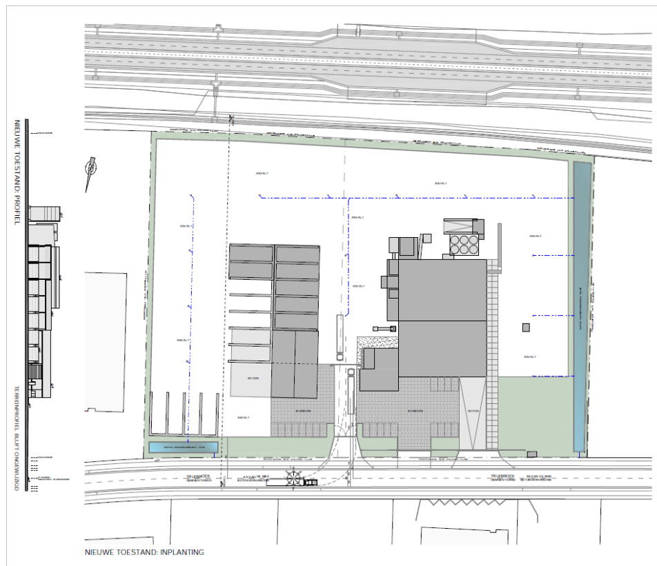
Figuur 2: Inplantingsplan geplande toestand (opdrachtgever, 2021)
