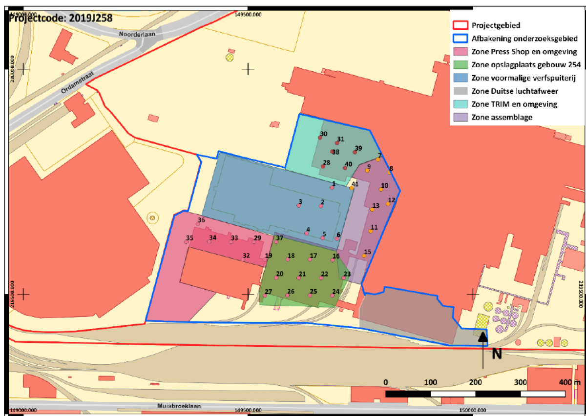
Figuur 14. Overzicht van de vijf onderzoekszones en de uitgevoerde landschappelijke boringen. (VERVOORT, 2020b, p. 19)
