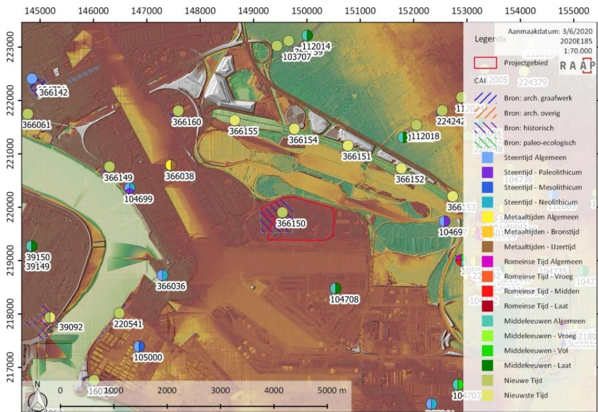
Figuur 13. Projectie van de betrokken percelen, de waterlopen en CAI-items op het digitaal terreinmodel Vlaanderen en de GRB-kaart (bron: AGIV, 2015, 2021; ONROEREND ERFGOED, 2018).
