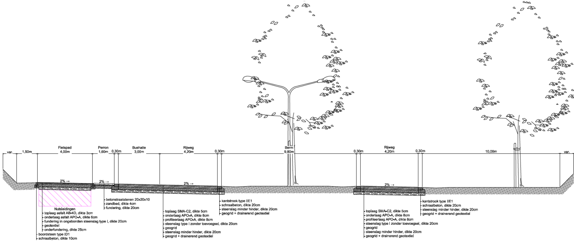
Typedwarsprofiel 1 1:100
