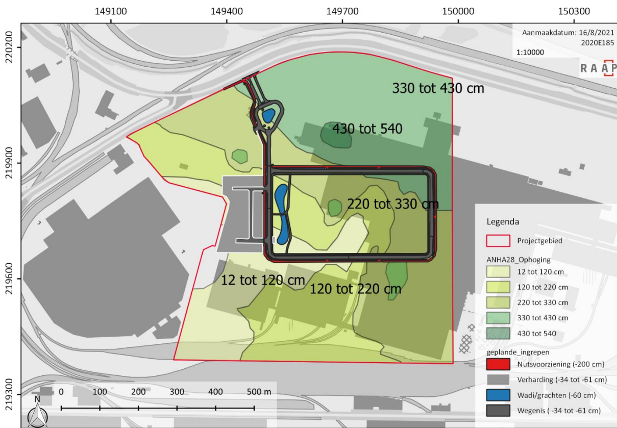
Figuur 10. Herwerkt opspuitingsmodel: dikte opspuitingen binnen de betrokken percelen op het moment van de sloop. (bron: o.b.v. VERVOORT, 2017, p. 101).
