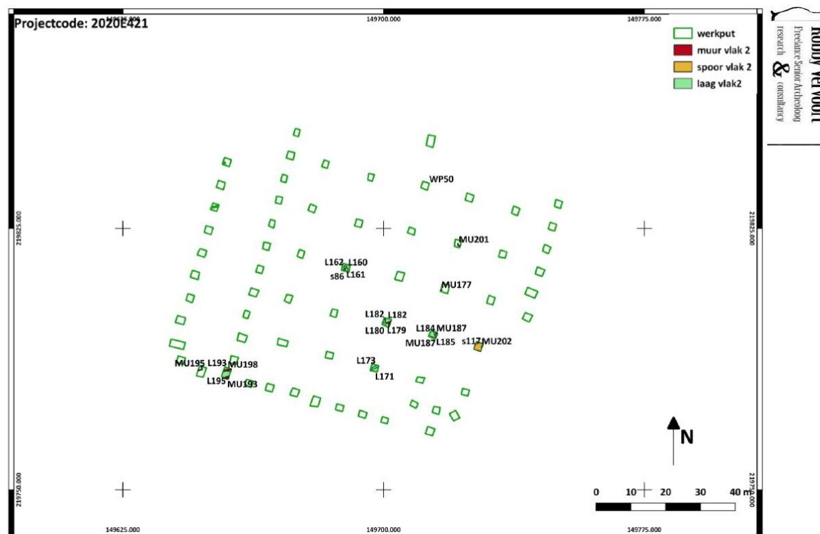
Figuur 22: overzicht aangetroffen sporen binnen vlak 1 van de zone "TRIM-Magezijn". (VERVOORT, 2020a)
