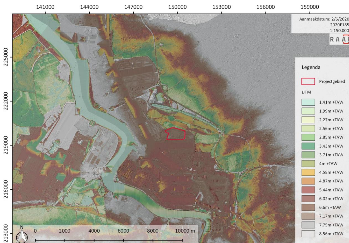
Figuur 11. Digitaal Terrein model Vlaanderen met aanduiding van het plangebied (rood) en de waterlopen (bron: AGIV, 2015; VMM, 2021).
