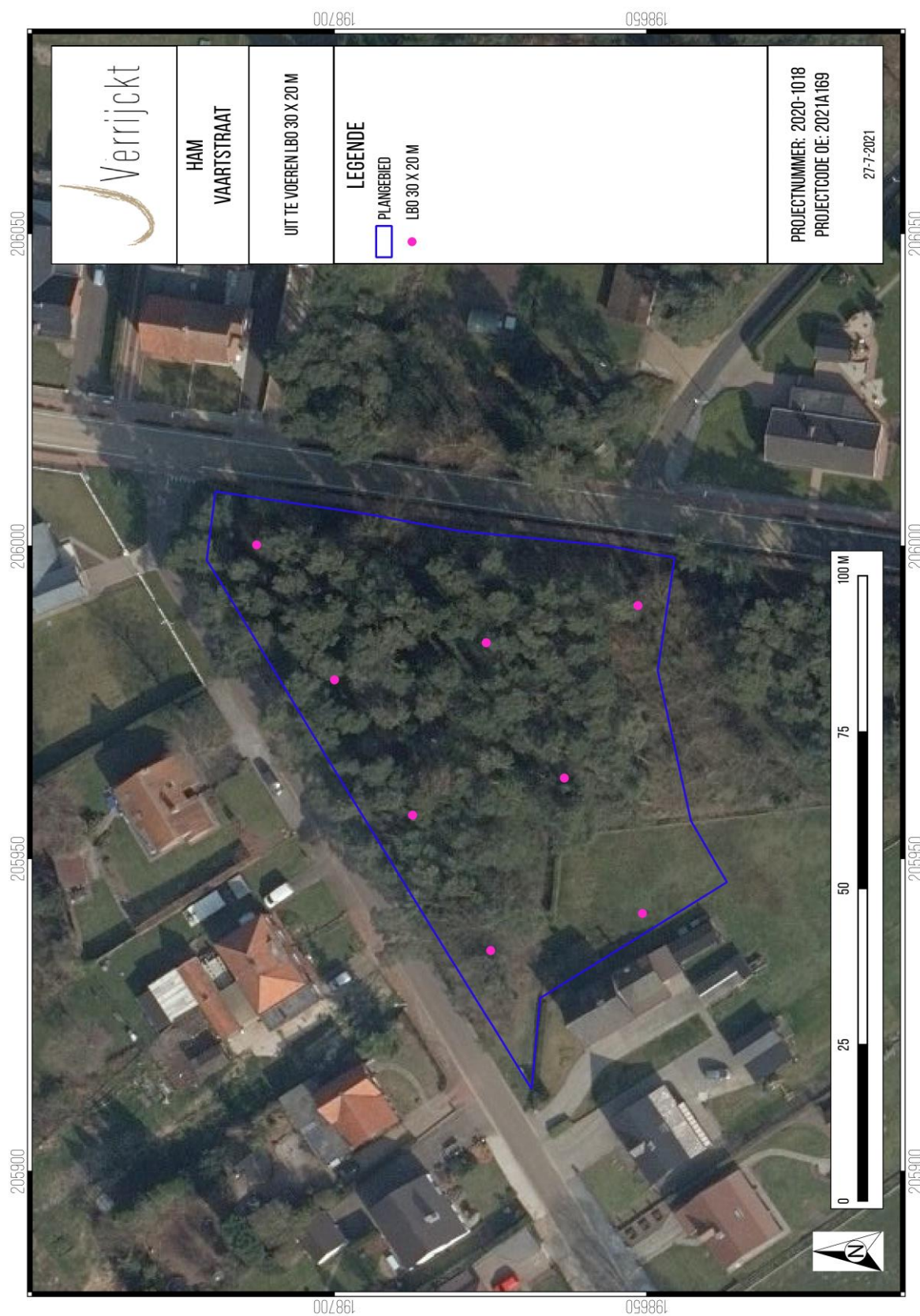
Figuur 2: Inplanting landschappelijke boringen op orthofoto 2
