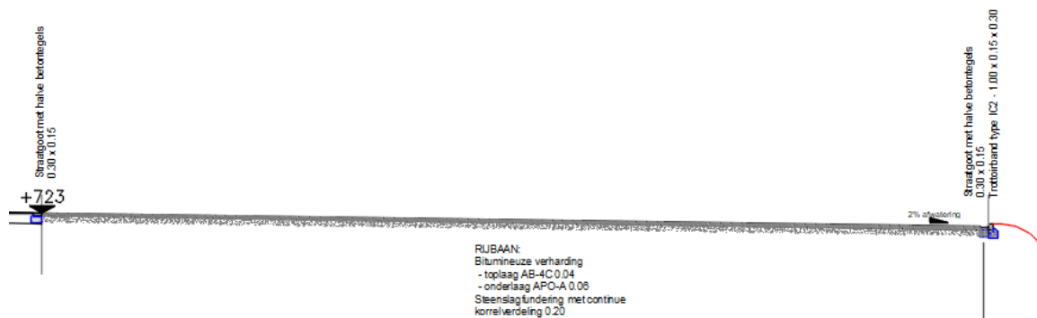
Figuur 7. Doorsnede van de toekomstige verharding (bron: opdrachtgever).
