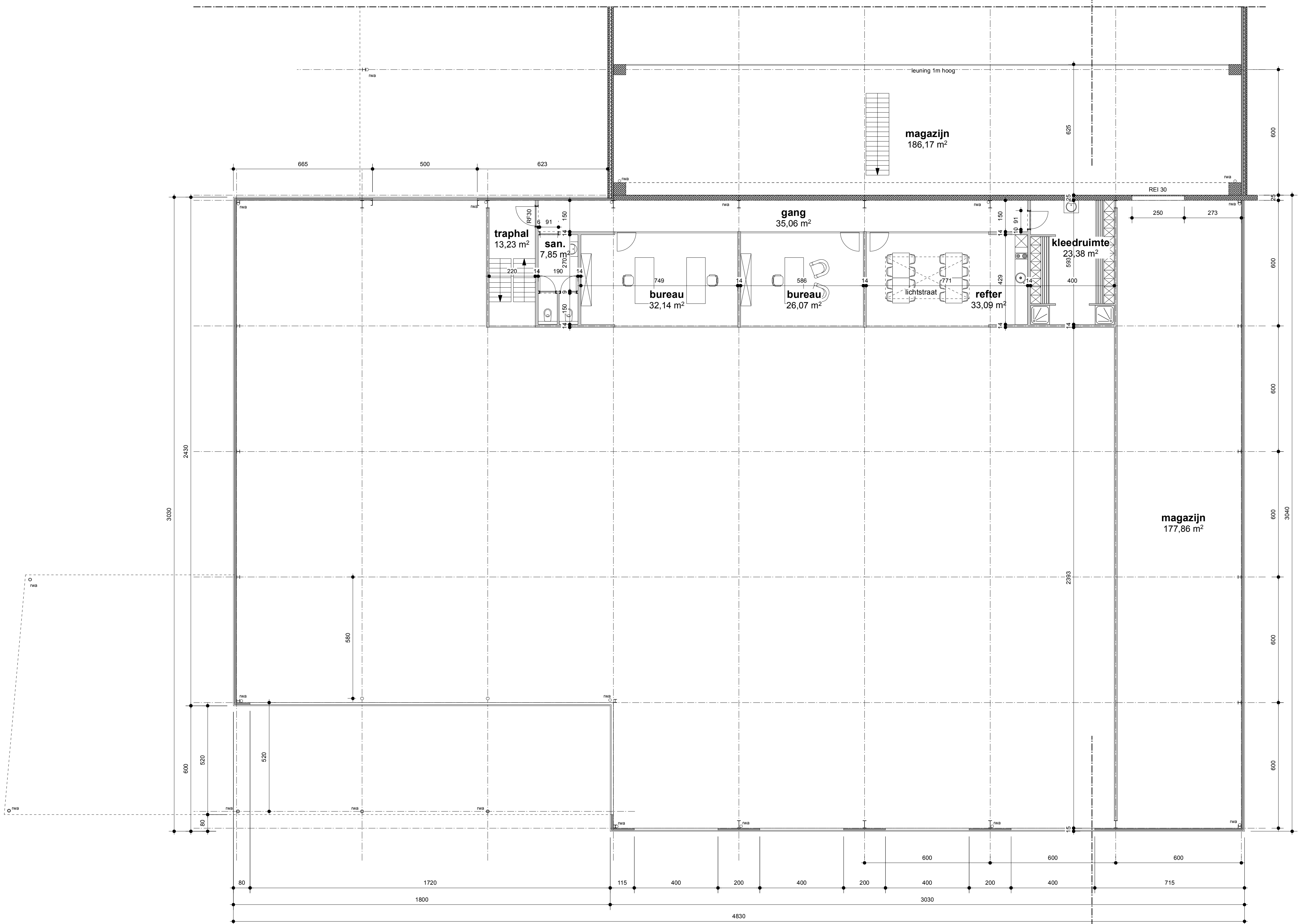
VERDIEPING 1 - GEBOUW 1
