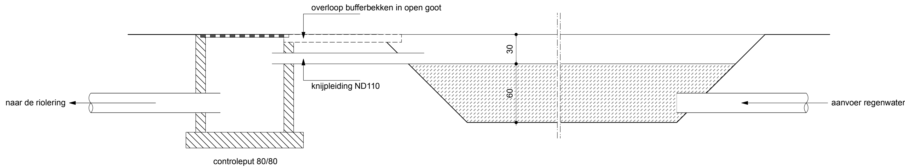
DETAIL - PRINCIPESNEDE BUFFERBEKKEN SCHAAL 1/20
