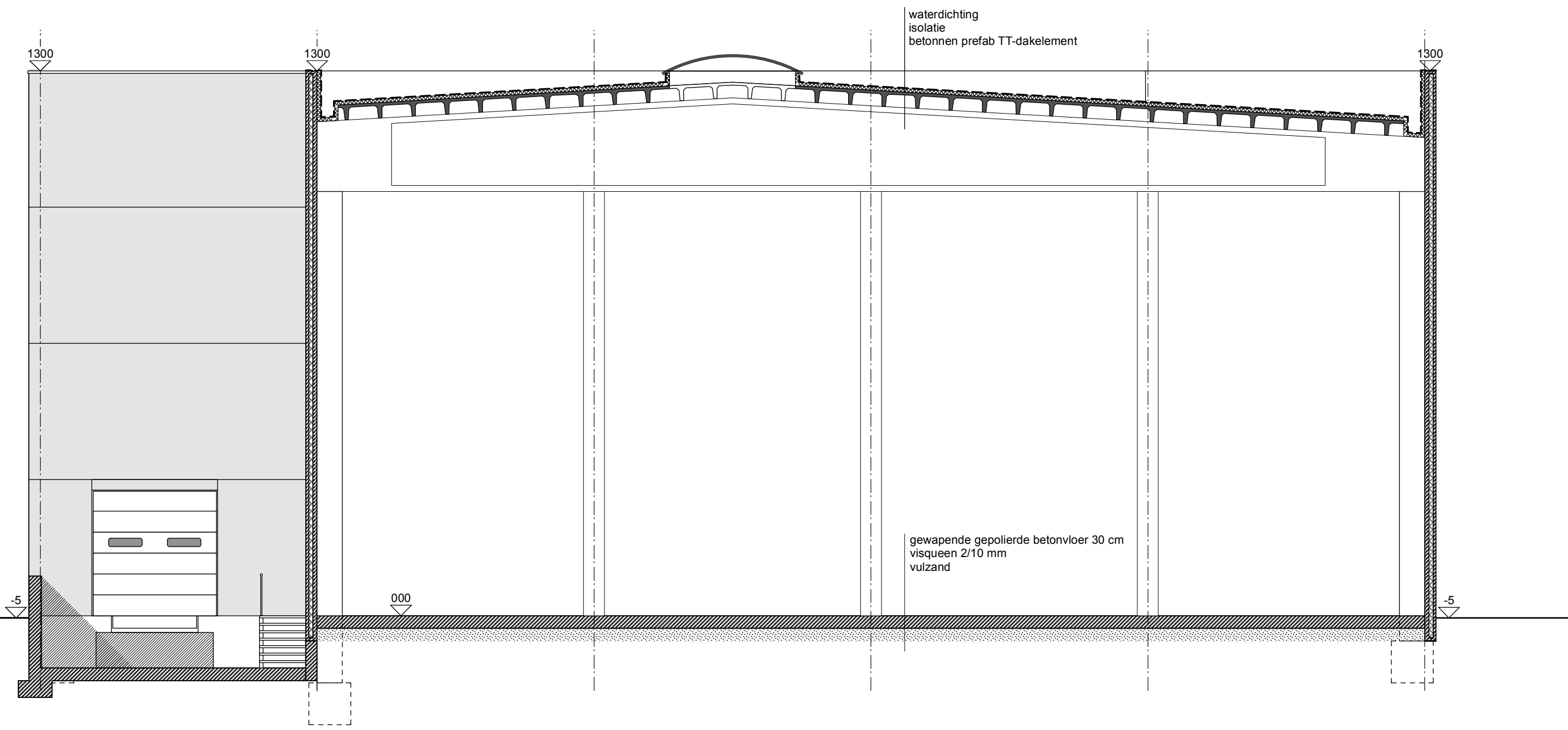
SNEDE B - GEBOUW 2 SCHAAL 1/100
