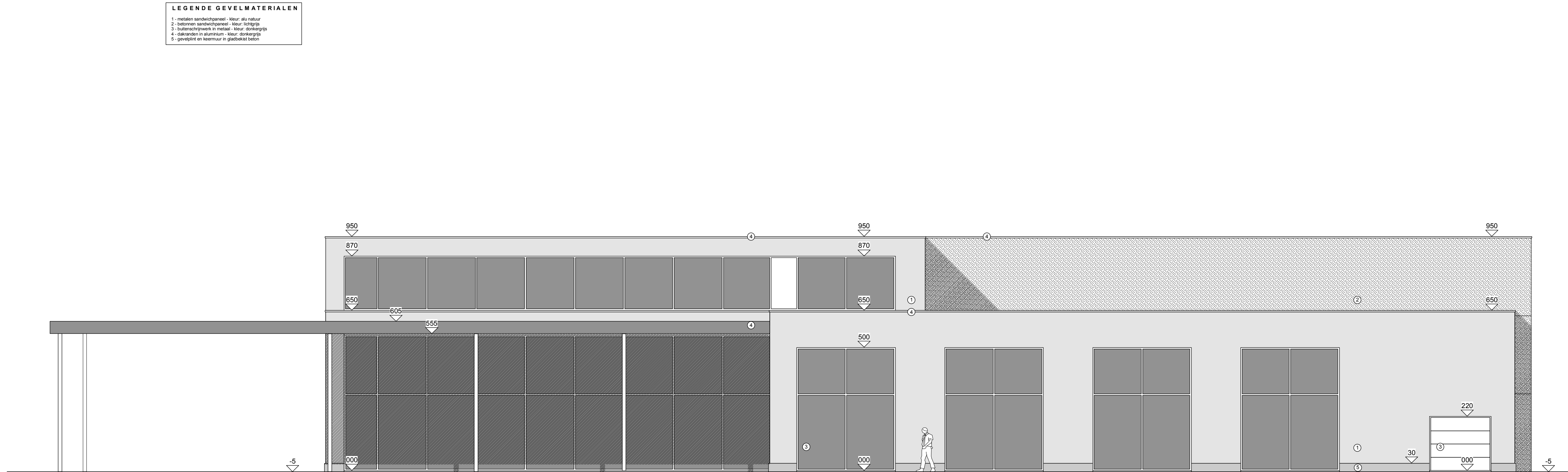
VOORGEVEL - GEBOUW 1 SCHAAL 1/100
