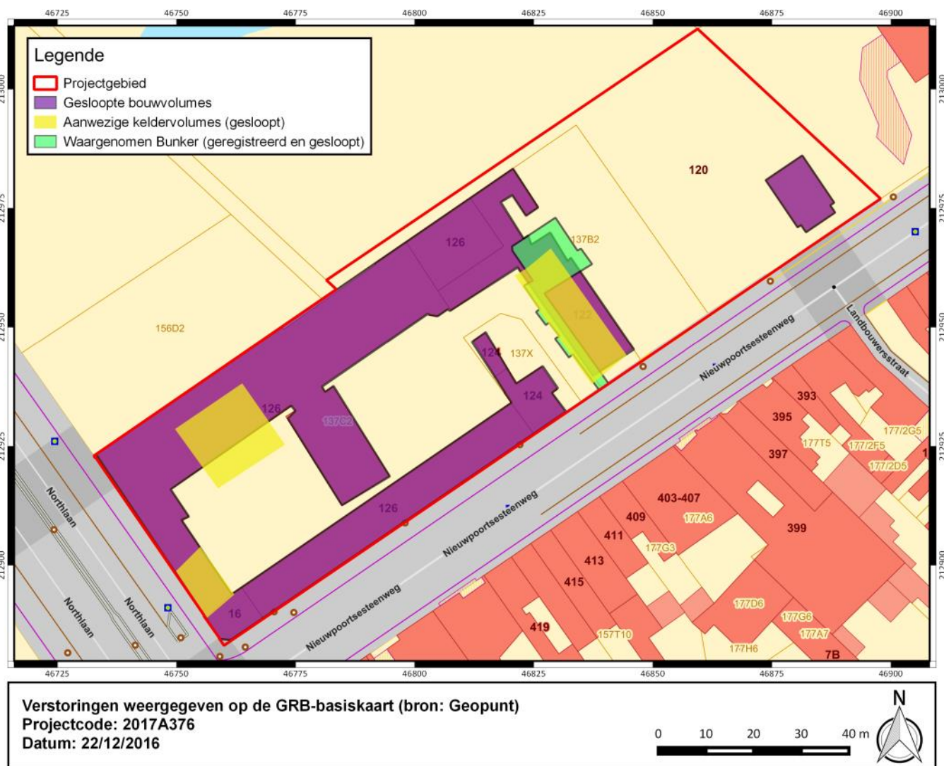
Figuur 3: verstoringskaart.
