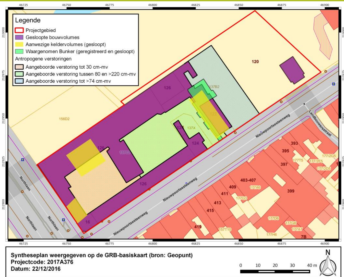
Figuur 27: syntheseplan.
