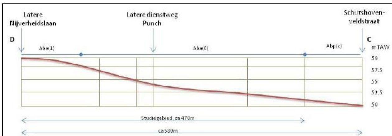
Afbeelding 7: Reconstructie van de oorspronkelijke topografie van het terrein
