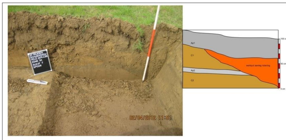
Afbeelding 12: profiel 2: kopprofiel noordzijde sleuf 7
