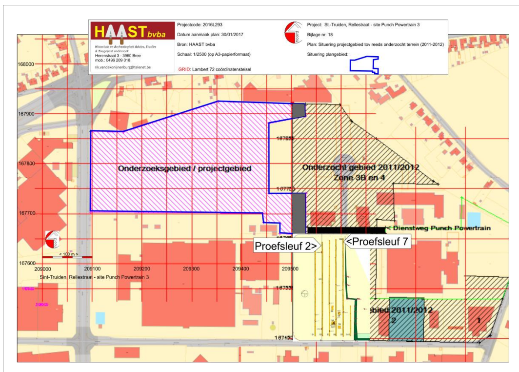
Afbeelding 13: situering van de proefsleuven 2 en 7 ten opzichte van het huidige projectgebied
