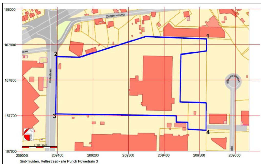
Afbeelding1: Bounding Box
