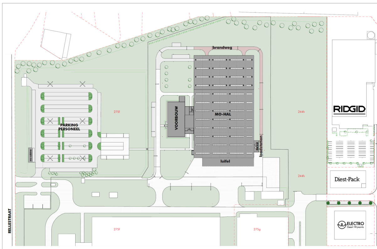
Afbeelding 4: inplanting nieuwbouw, verbouwingen, nieuwe aanleg (rood omkaderd de zones waar ingrepen in de bodem zullen gebeuren).
