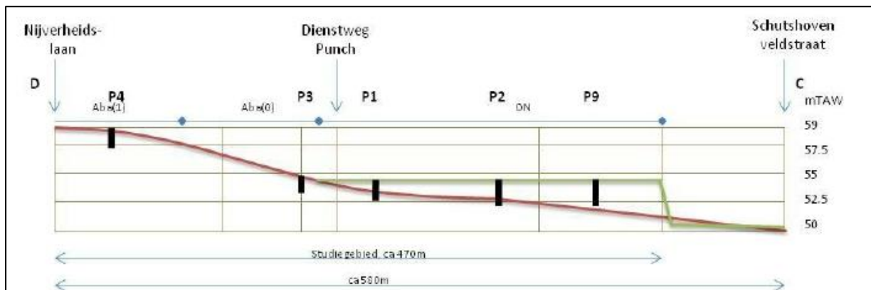
Afbeelding 8: huidige topografie van het terrein: Groen: huidige maaiveldhoogte ten noorden van de Dienstweg Punch, ophoging t.o.v. de oorspronkelijke topografie, P1 – P9: situering van de proefputten en boringen.
