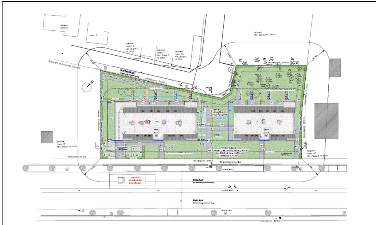
Figuur 3a. Inplantingsplan nieuwe toestand.
