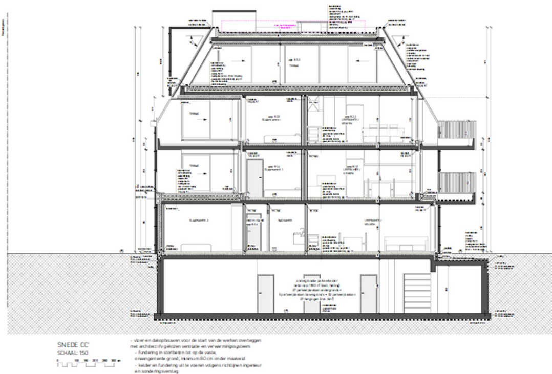
Figuur 3c. Doorsnedes.
