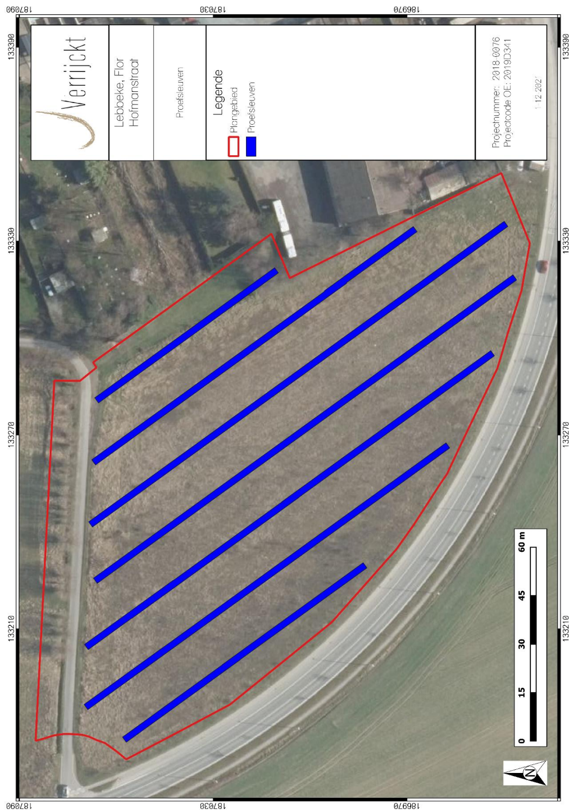
Figuur 3: Sleuvenplan weergegeven op GRB-basiskaart
