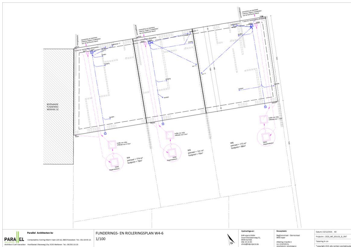
Figuur 10 Funderings- en rioleringsplan loten 4-6. (bron: opdrachtgever)
