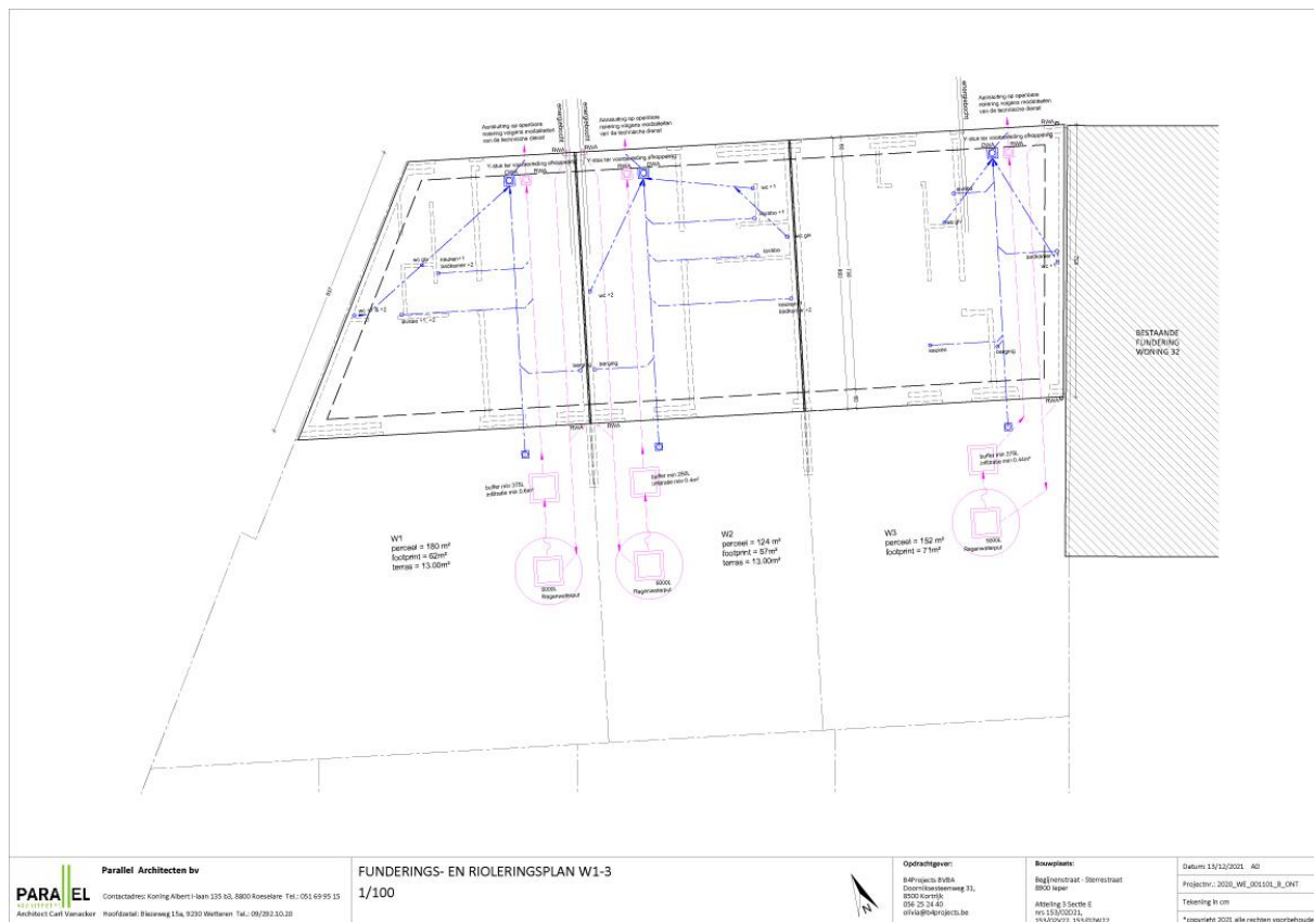
Figuur 9 Funderings- en rioleringsplan loten 1-3. (bron: opdrachtgever)
