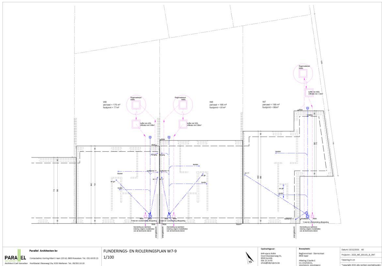
Figuur 11 Funderings- en rioleringsplan loten 7-9 . (bron: opdrachtgever)
