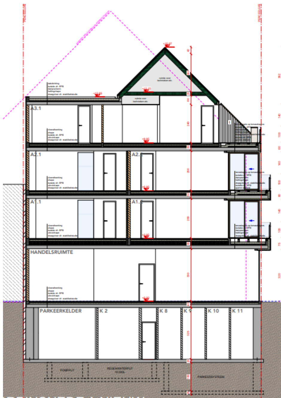
Figuur 11 Ontwerpplan - snede (initiatiefnemer, 2022)
