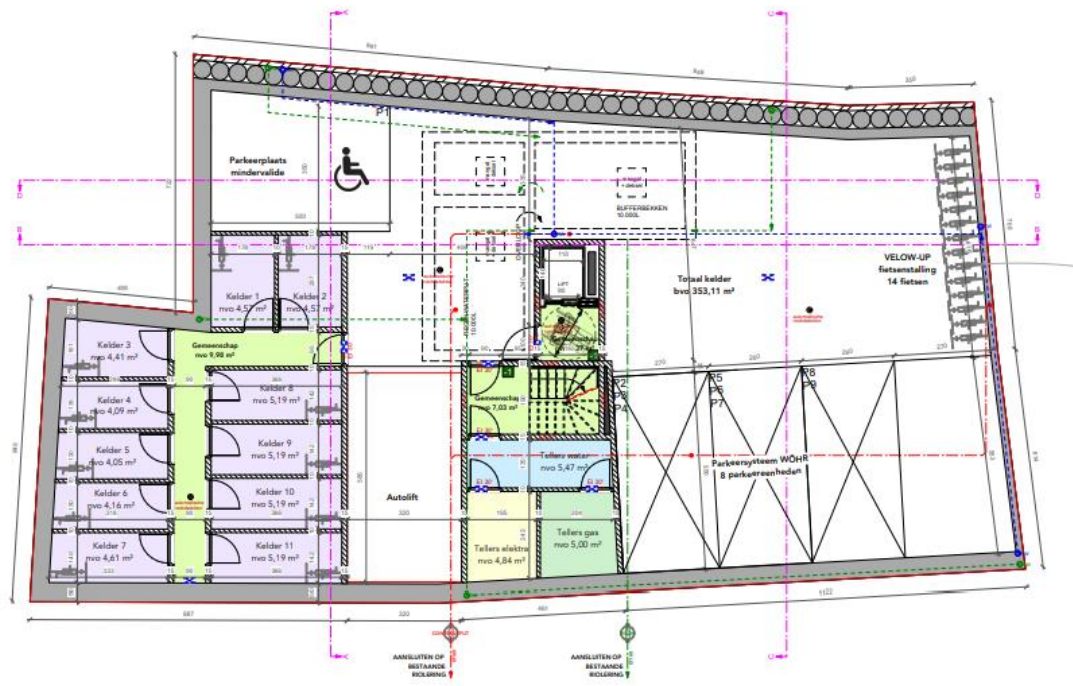
Figuur 9: ontwerpplan – kelderniveau (initiatiefnemer, 2022).
