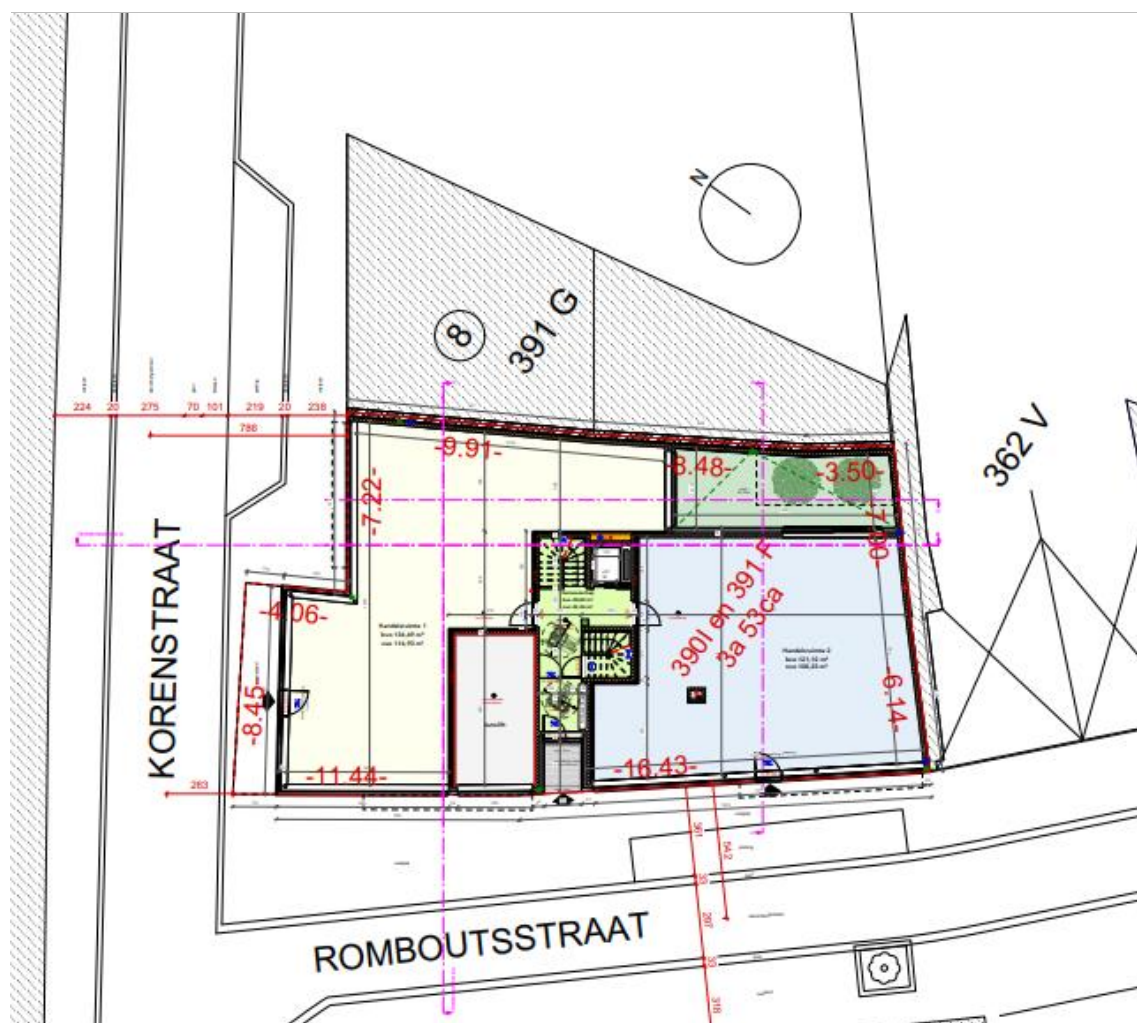
Figuur 8: ontwerpplan - gelijkvloers (initiatiefnemer, 2022).
