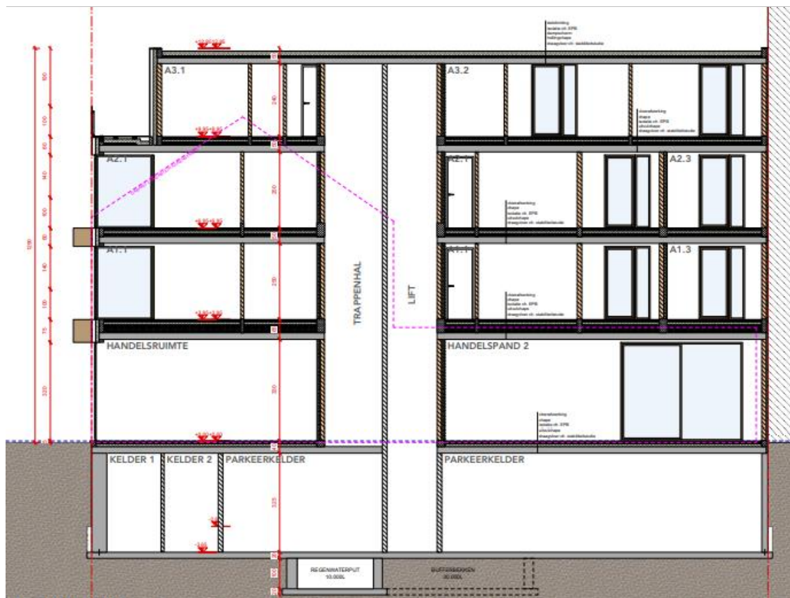
Figuur 10: Ontwerpplan - snede (initiatiefnemer, 2022)
