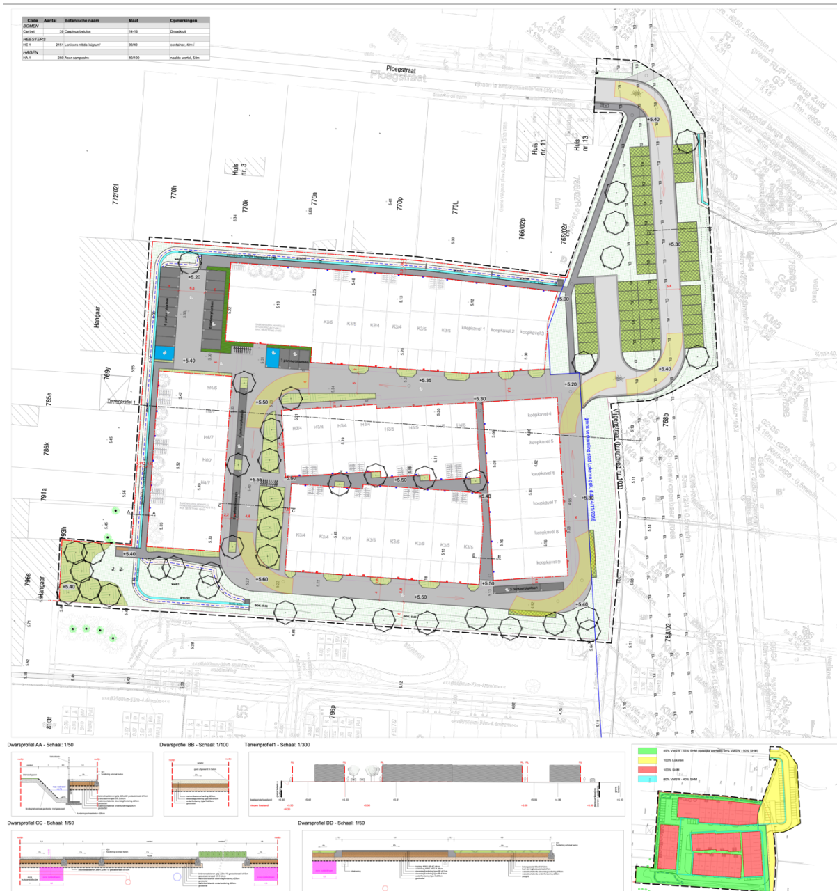
Fig. 3.4: Bouwplan 16 .
