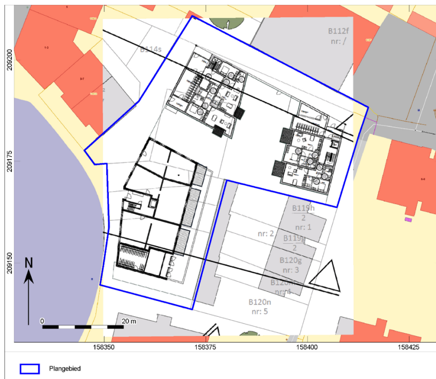
Fig. 1.1: Uitsnede van het inplantingsplan ter hoogte van deelgebied 3 (©VEC en initiatiefnemer).
