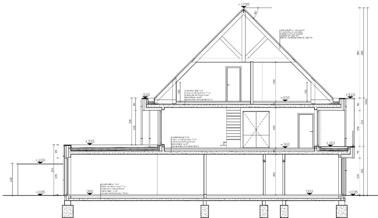
DOORSNEDE AA nieuwe toestand - duo-woning 5 SCHAAL 1/50
