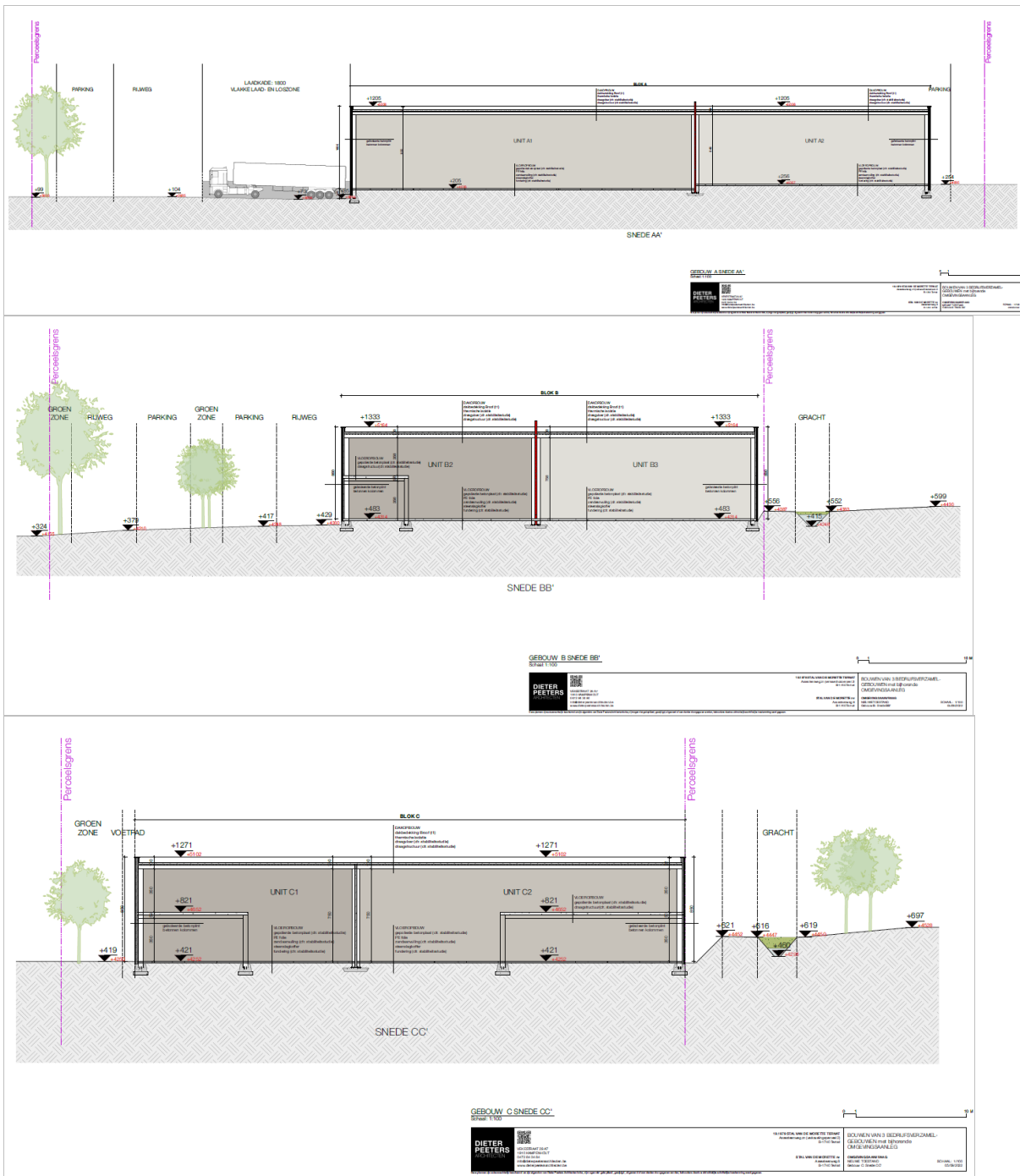
Figuur 10: Snedes (opdrachtgever, 2022)
