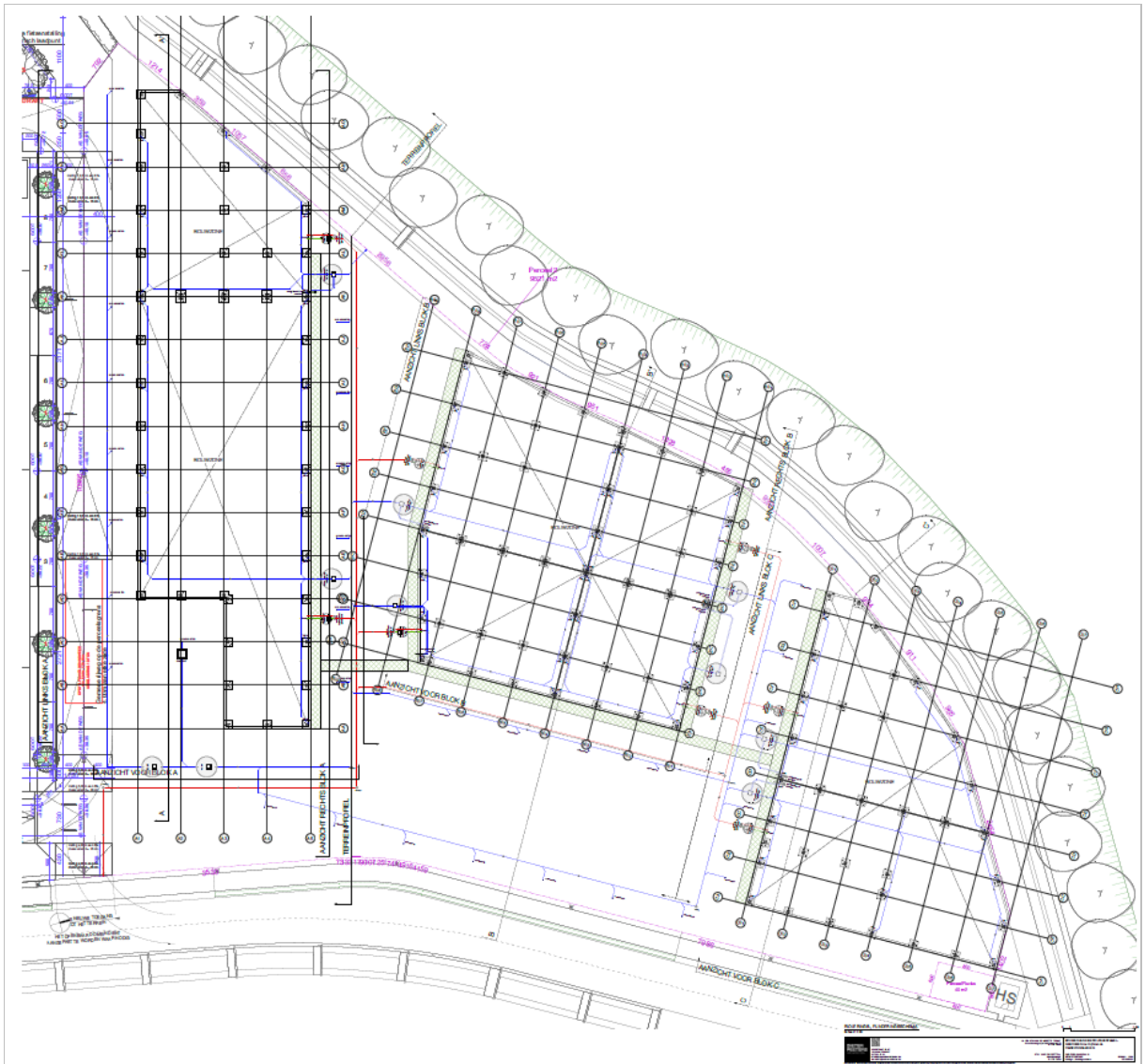
Figuur 9: Funderingsplan (opdrachtgever, 2022)
