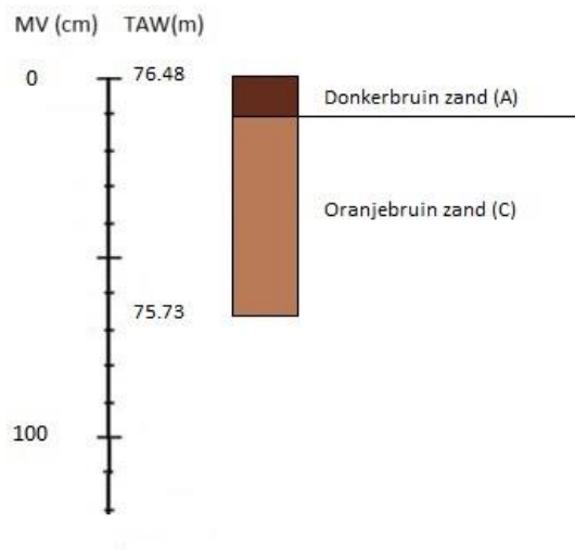
Figuur 14: Boorstaat B3 (Geopunt, 2022)
