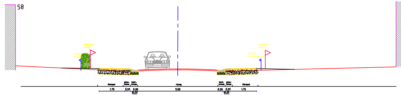
PROFIEL 2 zandstraat omgeving huish. 58
