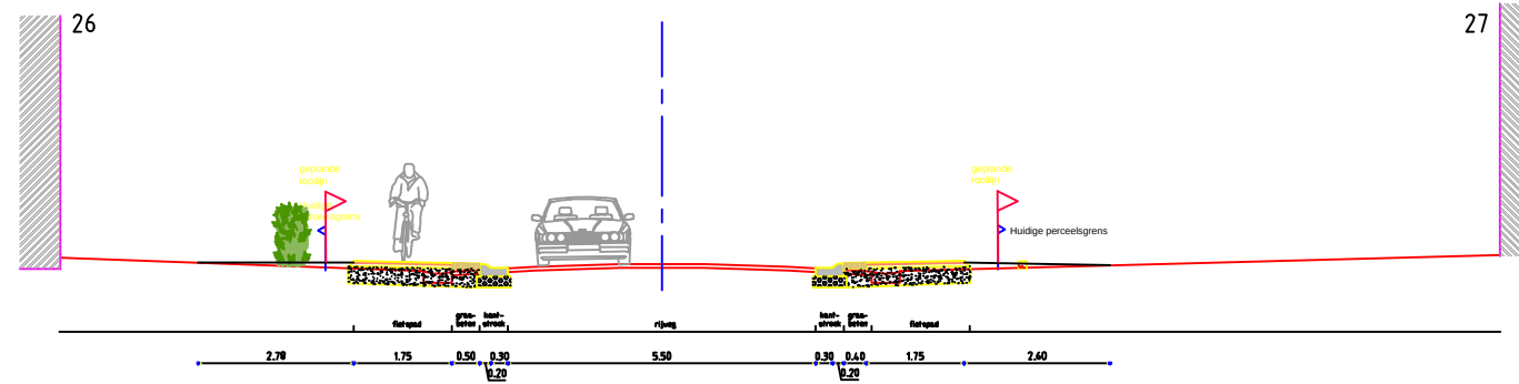
PROFIEL 1 zandstraat omgeving huish. 26
