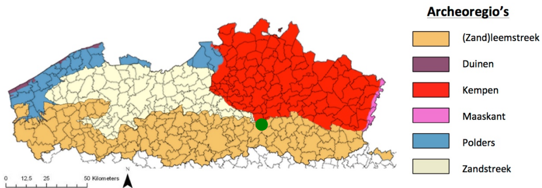
Fig. 3.1: Situering van het projectgebied binnen de verschillende Vlaamse archeoregio's 13 .
