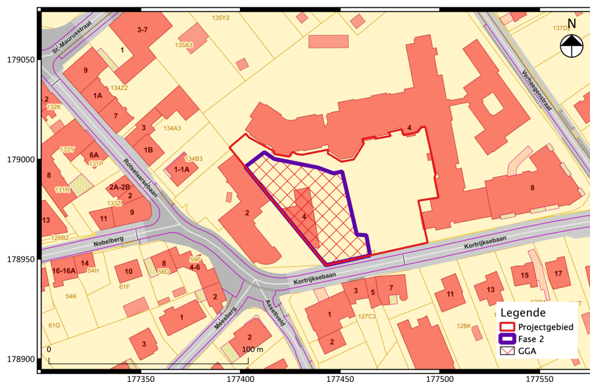
Fig. 3.3: Synthesekaart met zone die op de GGA-kaart mag worden opgenomen.
