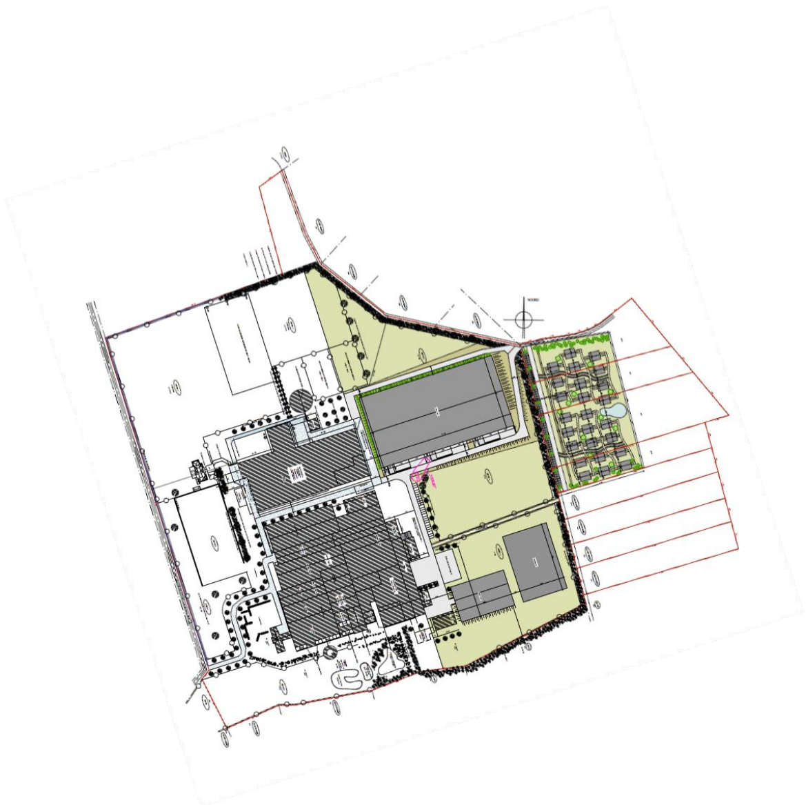
Figuur 3: Plan van de nieuwe toestand. (Opdrachtgever, 2023)
