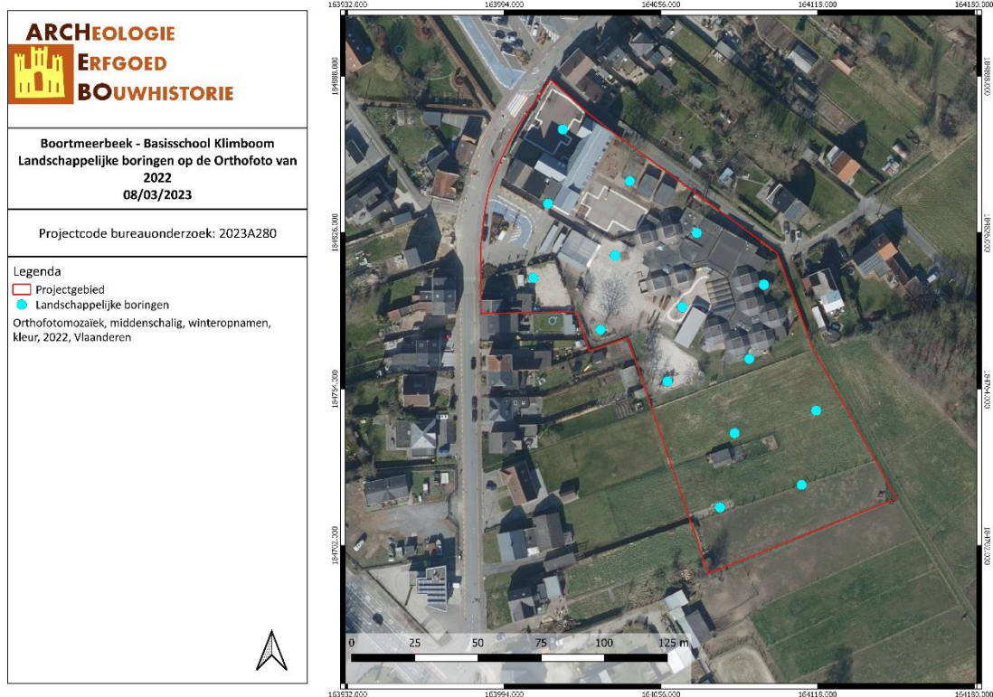
Figuur 5: Locatie boorpunten op het onderzoeksterrein (ARCHEBO bvba, 2023)
