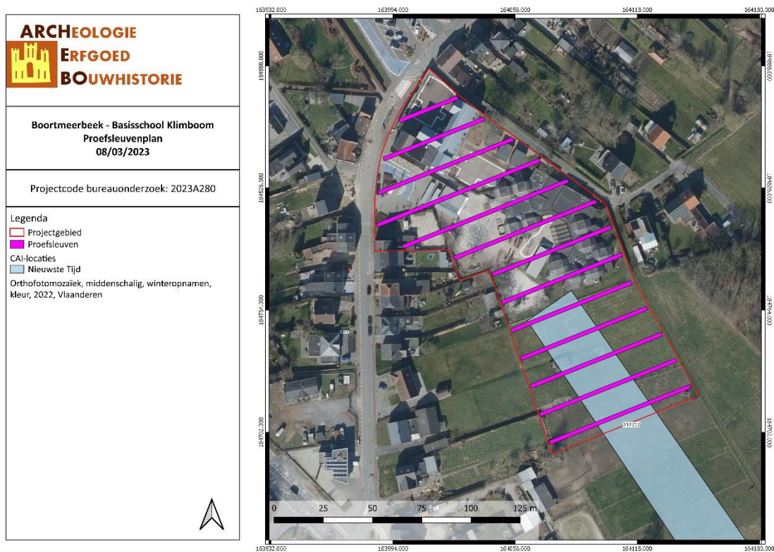
Figuur 6: Proefsleuven op het GRB (ARCHEBO bvba, 2023)
