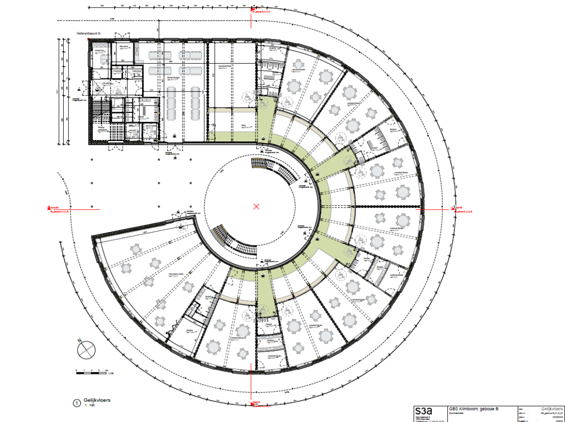
Figuur 4: Inplantingsplan gebouw B (Opdrachtgever, 2023)
