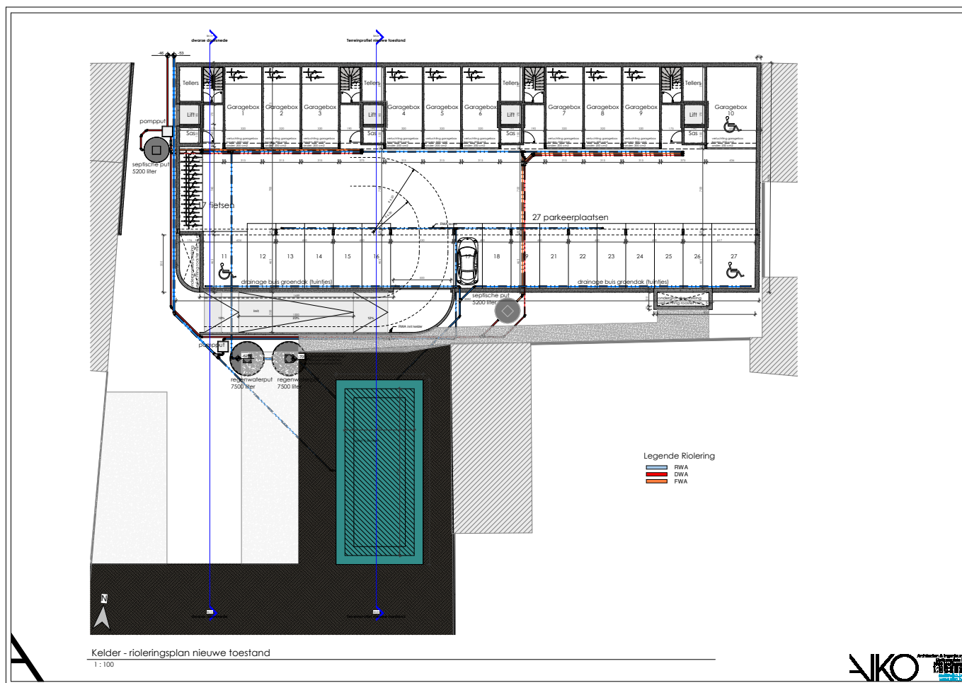
Figuur 6: Plan van de ondergrondse parking en rioleringsvoorziening (© AIKO Architecten & Ingenieurs)
