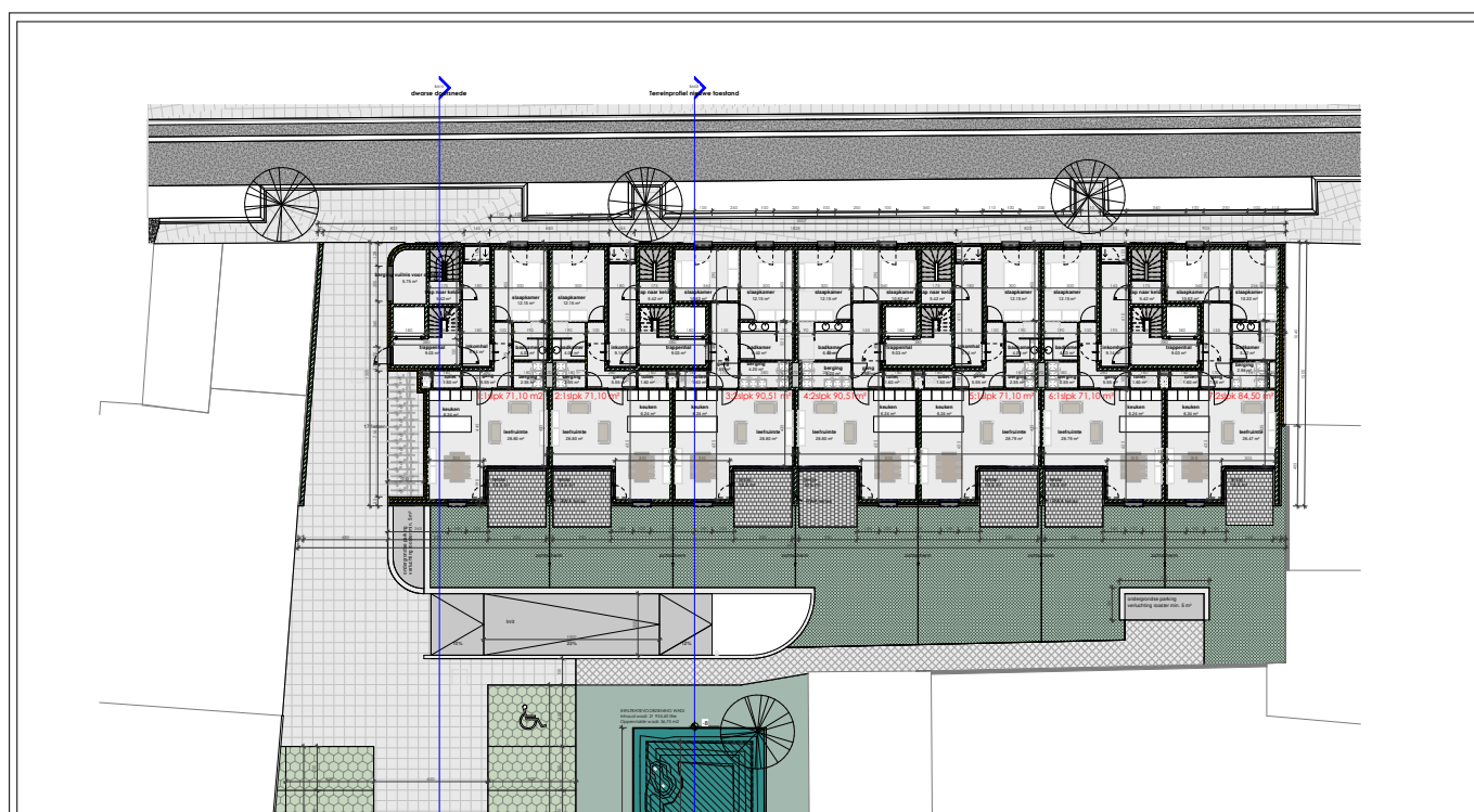
Figuur 7: Plan van het gelijkvloers niveau (© AIKO Architecten & Ingenieurs)
