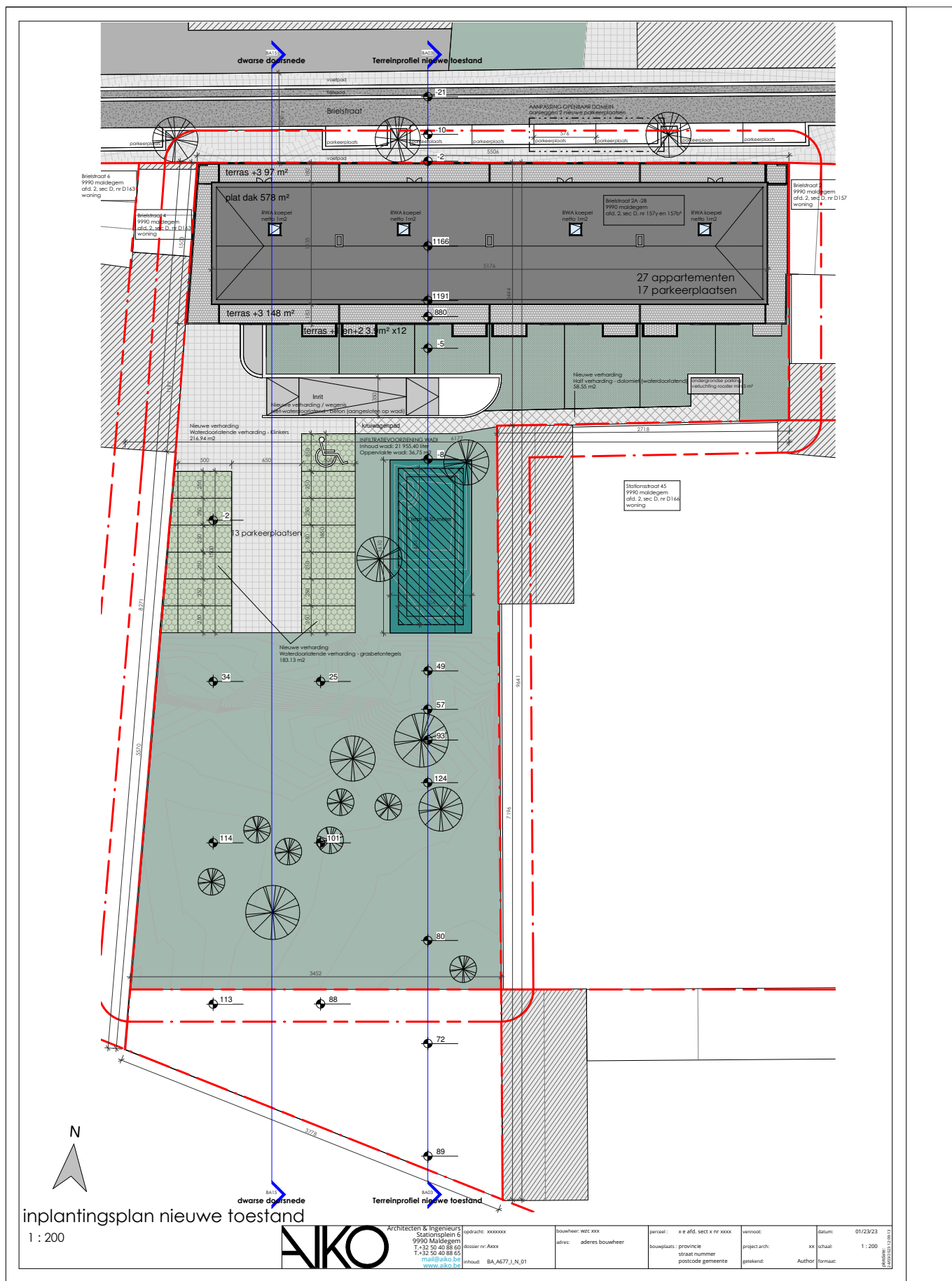
Figuur 3: Inplantingsplan van de nieuwe ontwikkeling (© AIKO Architecten & Ingenieurs)
