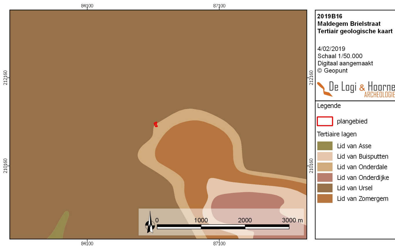
Figuur 10: Tertiair geologische kaart met aanduiding van het projectgebied (© Geopunt)
