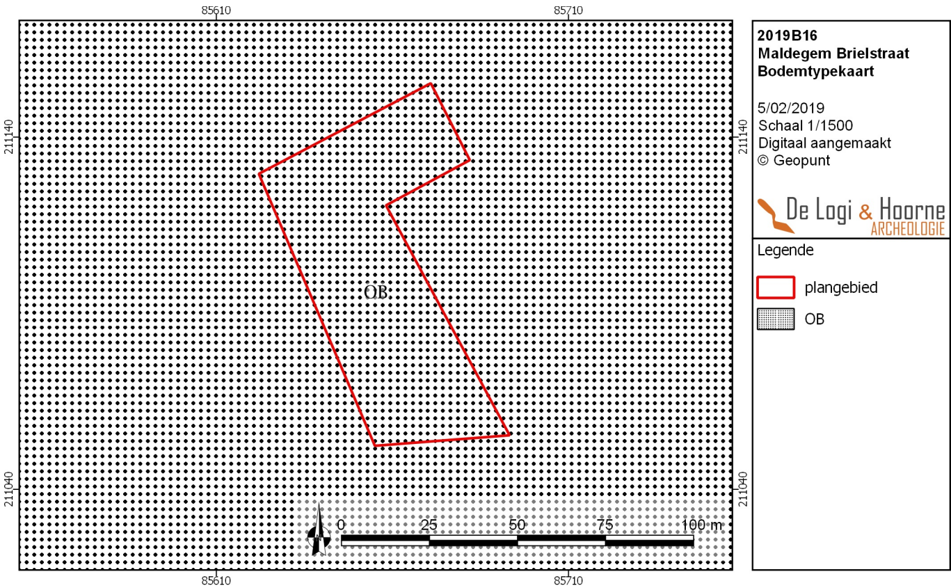
Figuur 12: Bodemtypekaart met aanduiding van het projectgebied (© Geopunt)
