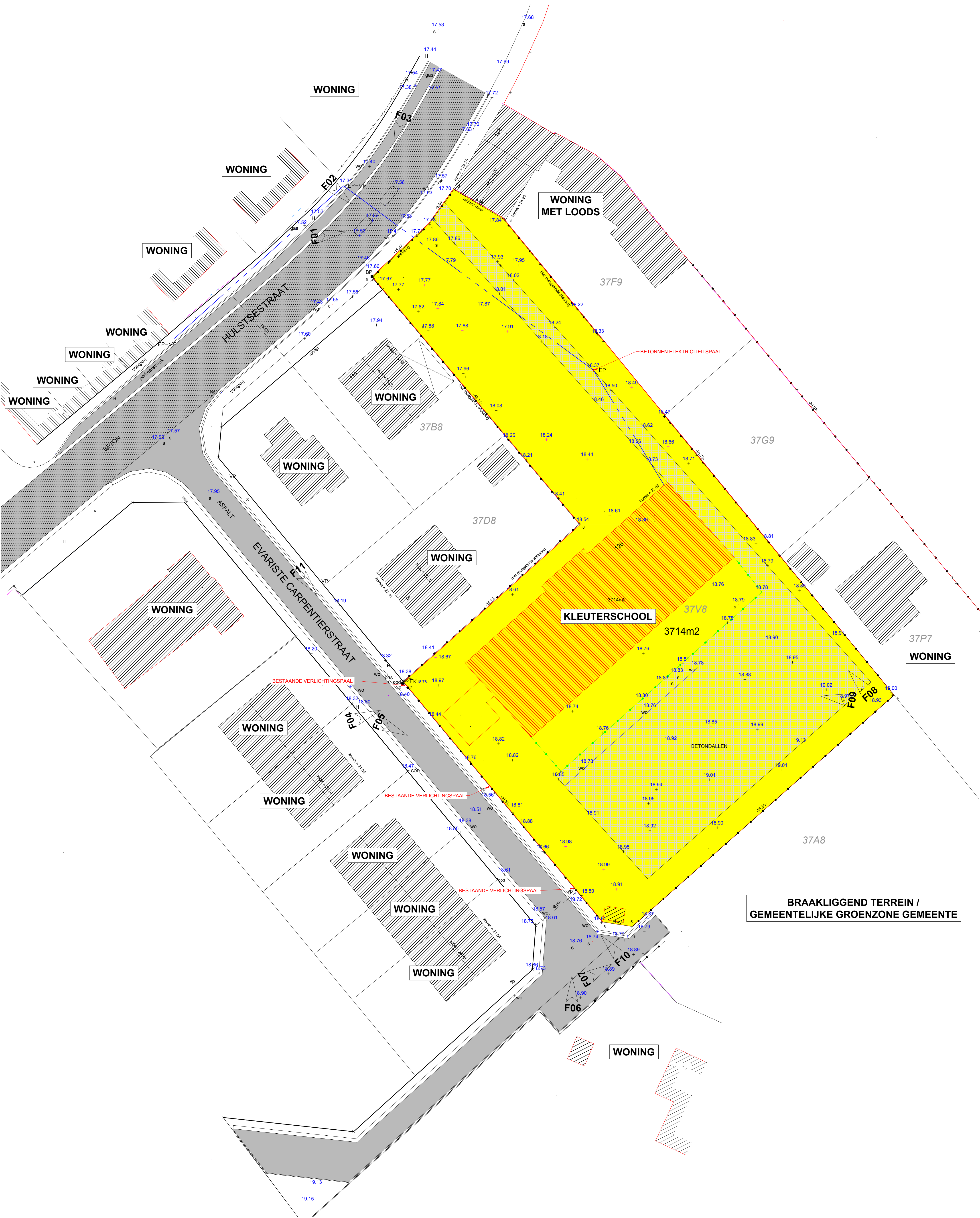
PLAN VERKAVELING BESTAANDE TOESTAND 1:250
