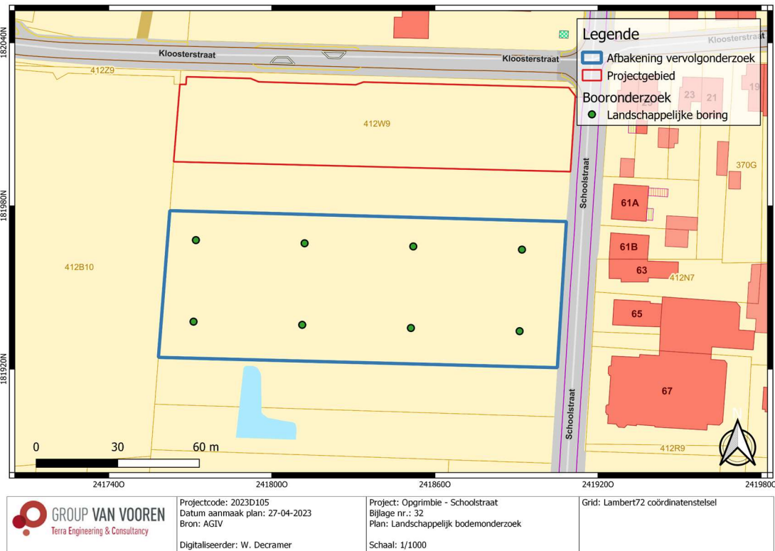
Fig. 2.6: Voorstel boorpuntenplan.
