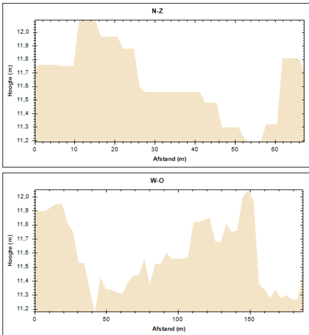
Figuur 9. Hoogteprofielen.
