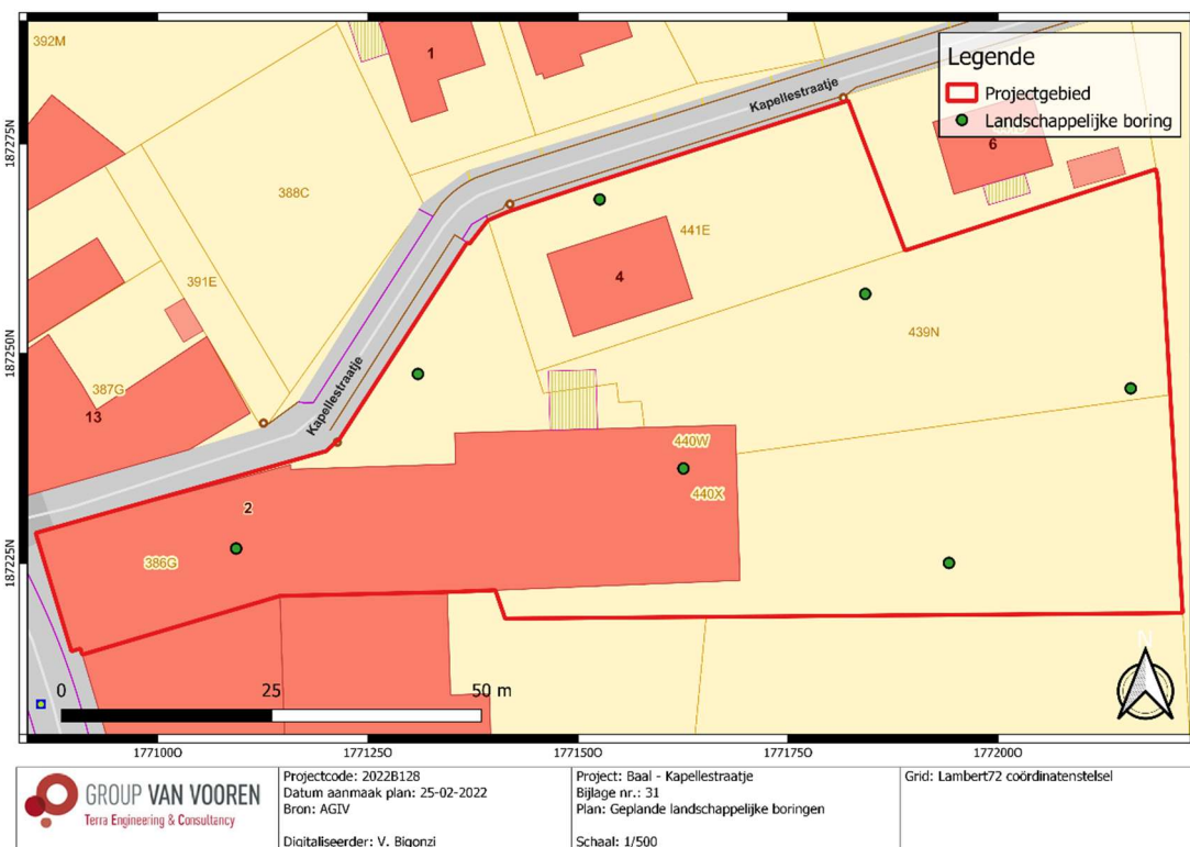
Fig. 2.5.: Voorstel boorpuntenplan.
