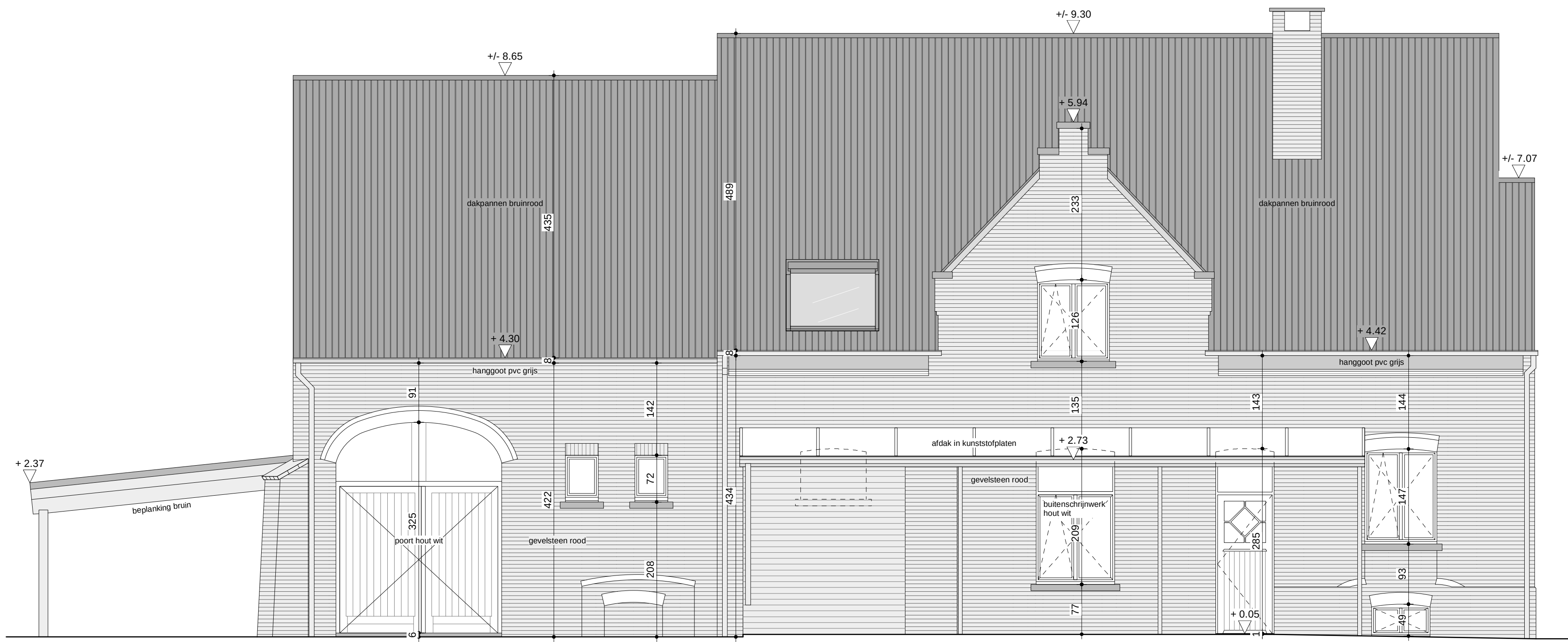
ACHTERGEVEL (NOORD) BESTAANDE TOESTAND - SCHAAL 1/50
