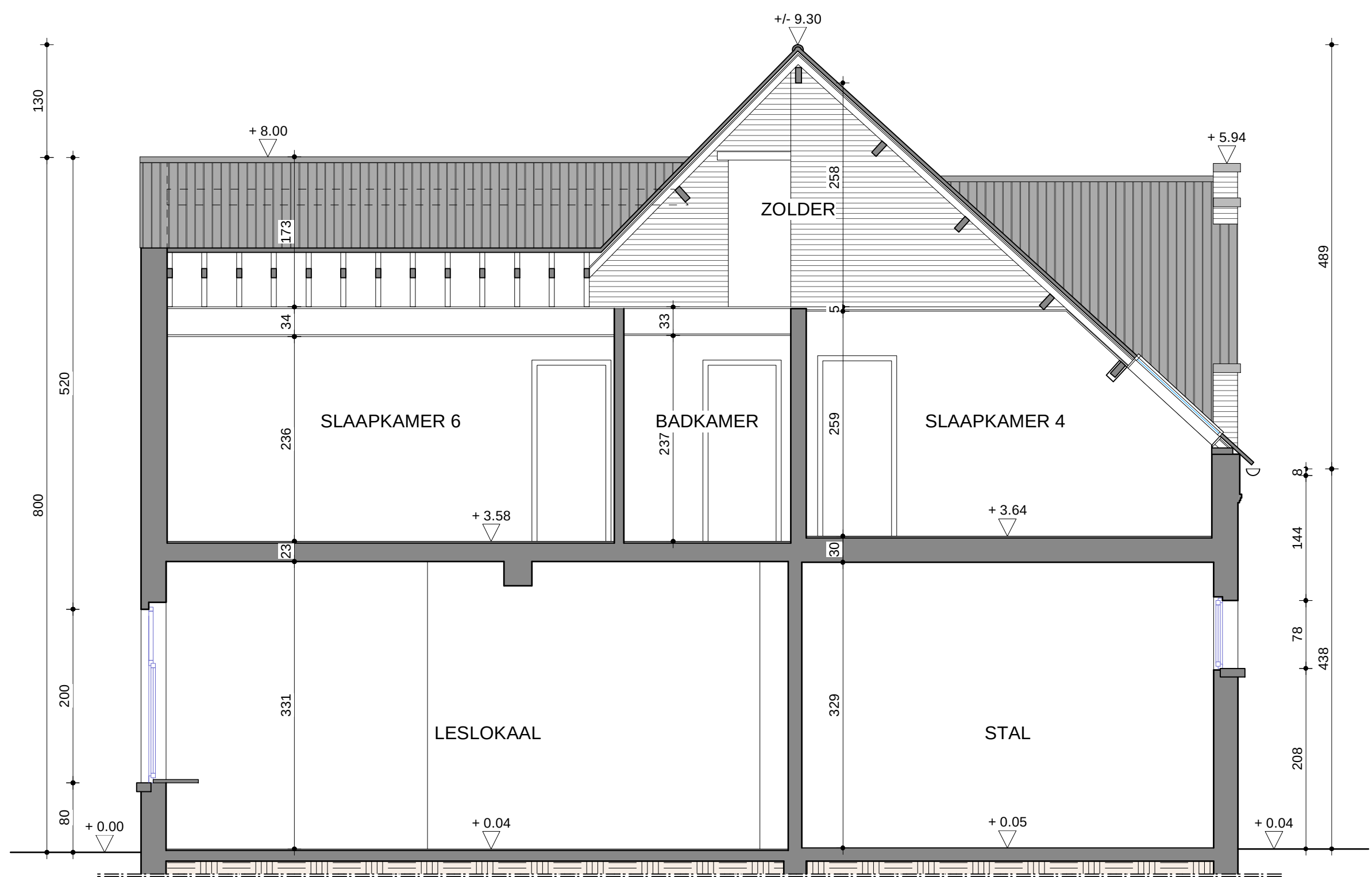
DOORSNEDE A-A' BESTAANDE TOESTAND - SCHAAL 1/50
