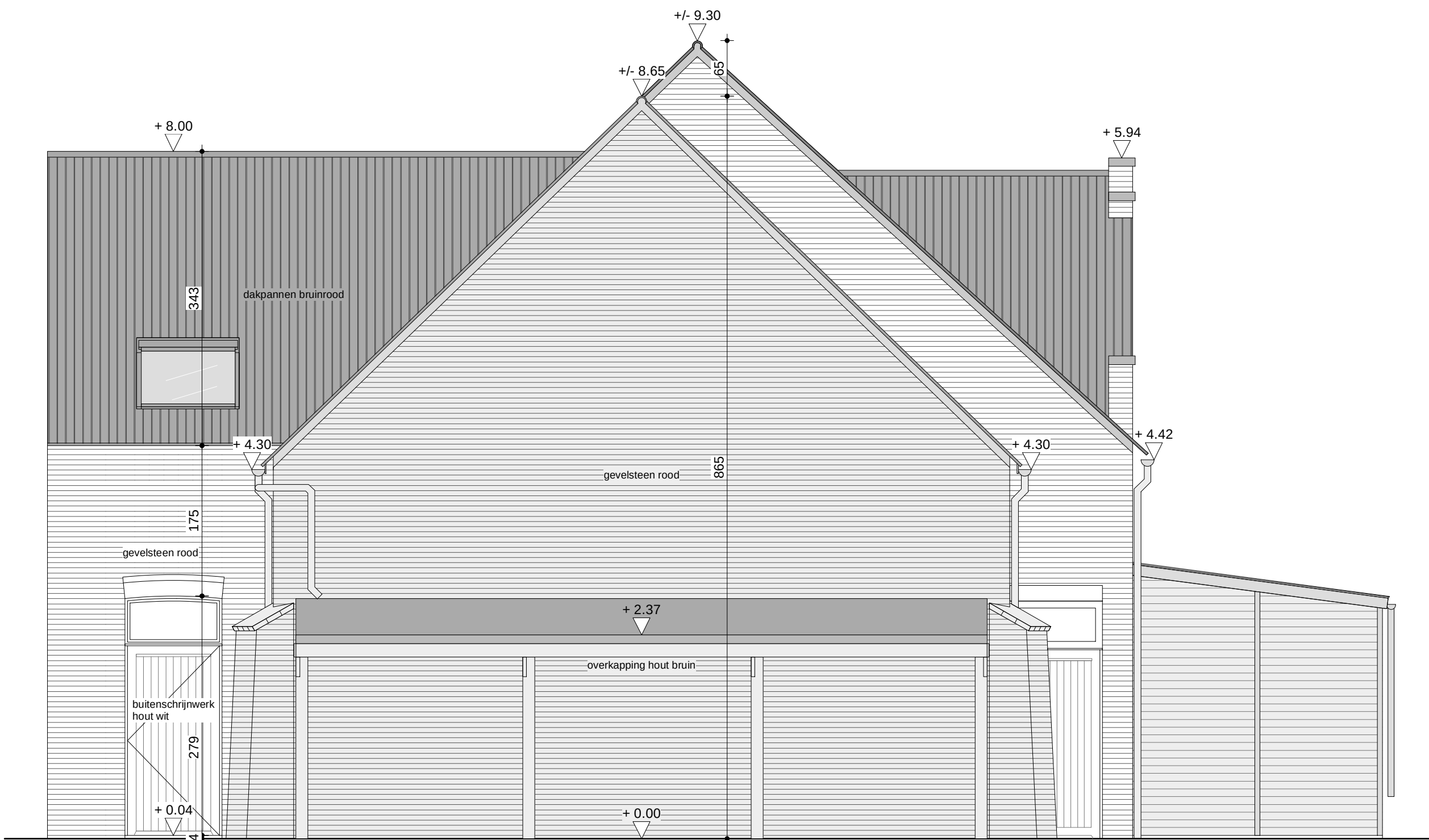
ZIJGEVEL RECHTS (OOST) BESTAANDE TOESTAND - SCHAAL 1/50
