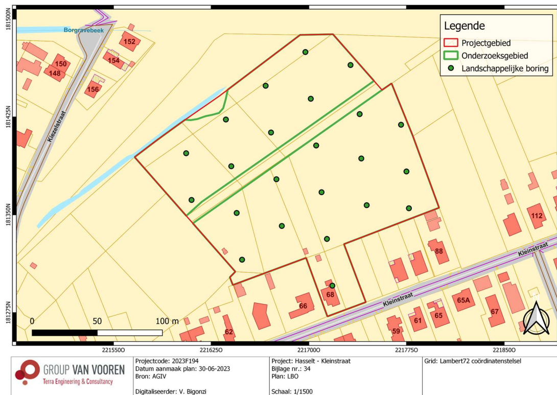
Fig. 2.7: Voorstel boorpuntenplan.
