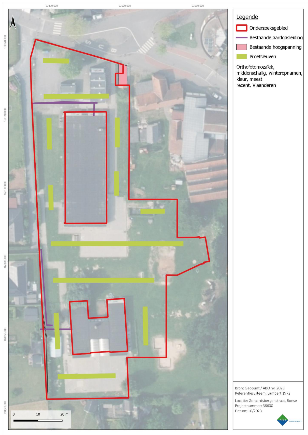
Figuur 42: Luchtfoto met indicatieve locatie van de proefsleuven.
