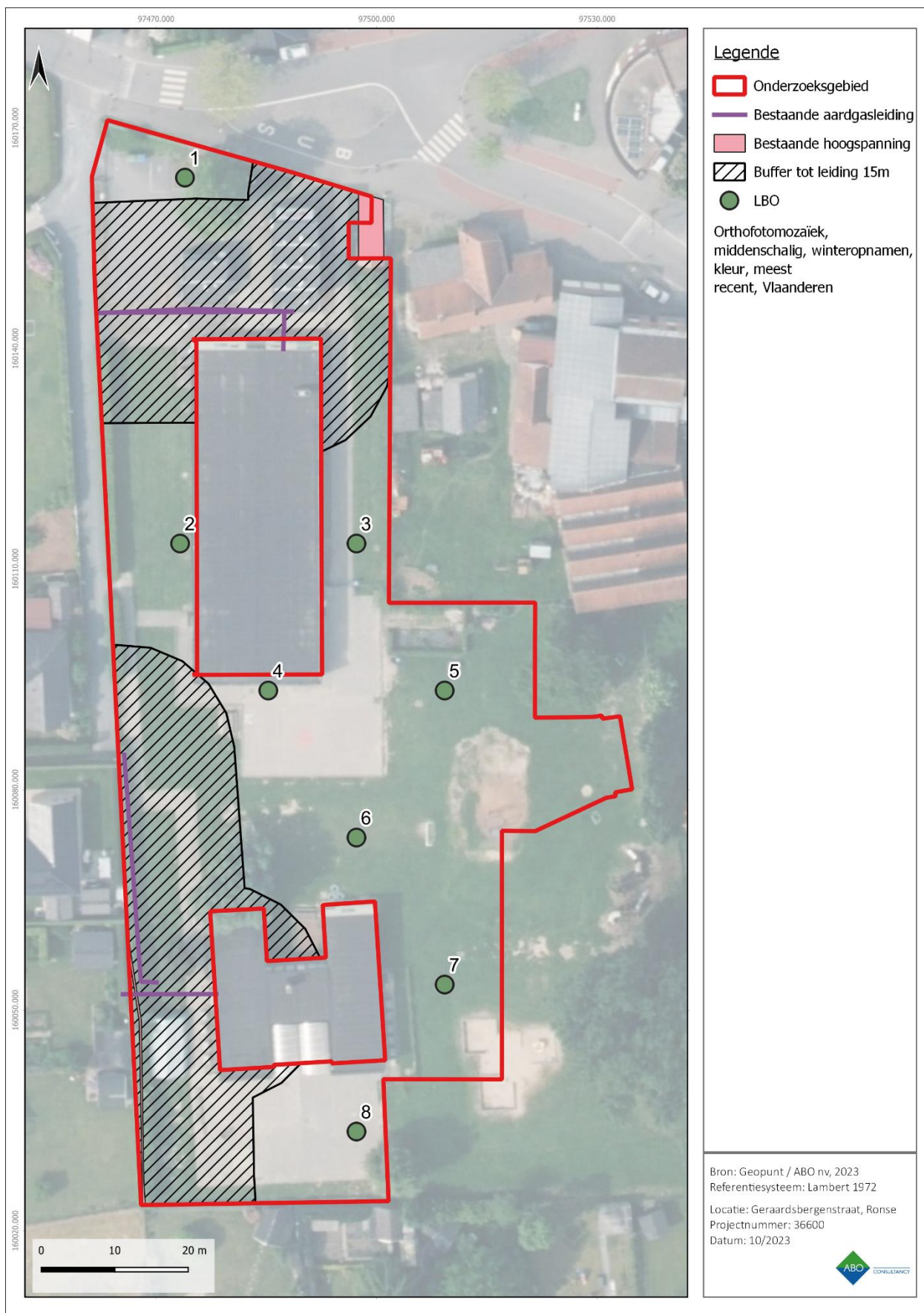
Figuur 41: Luchtfoto met aanduiding van de boorpunten voor het landschappelijk bodemonderzoek.
