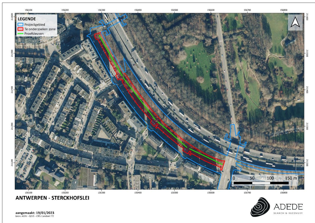
Figuur 3. Proefsleuvenplan
