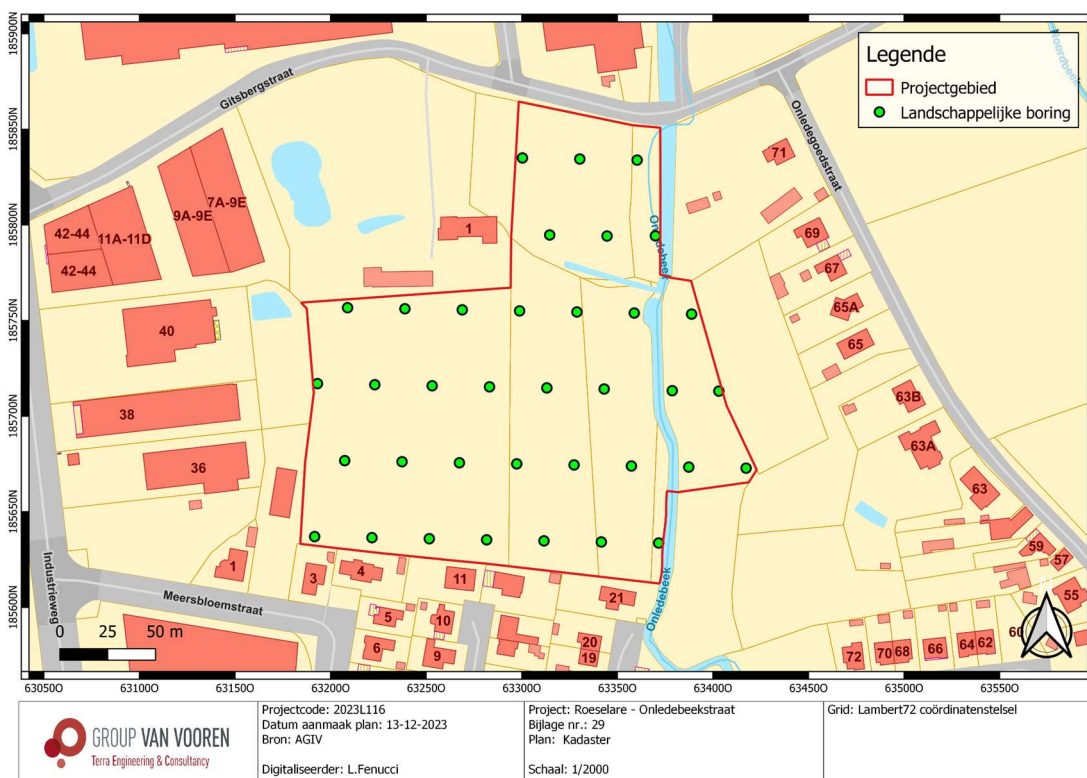
Fig. 2.5: Voorstel boorpuntenplan.
