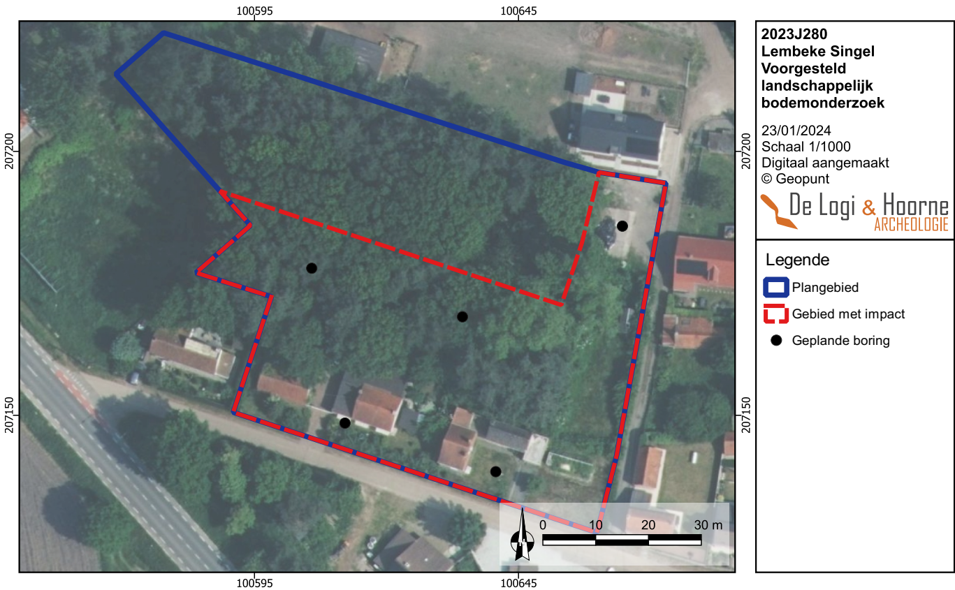
Figuur 22: De voorgestelde landschappelijke boringen geprojecteerd op een recente luchtfoto
