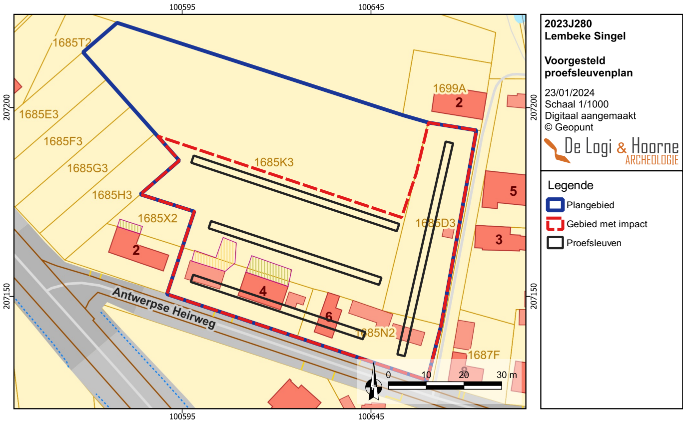
Figuur 23: Proefsleuvenschema weergegeven op het kadaster
