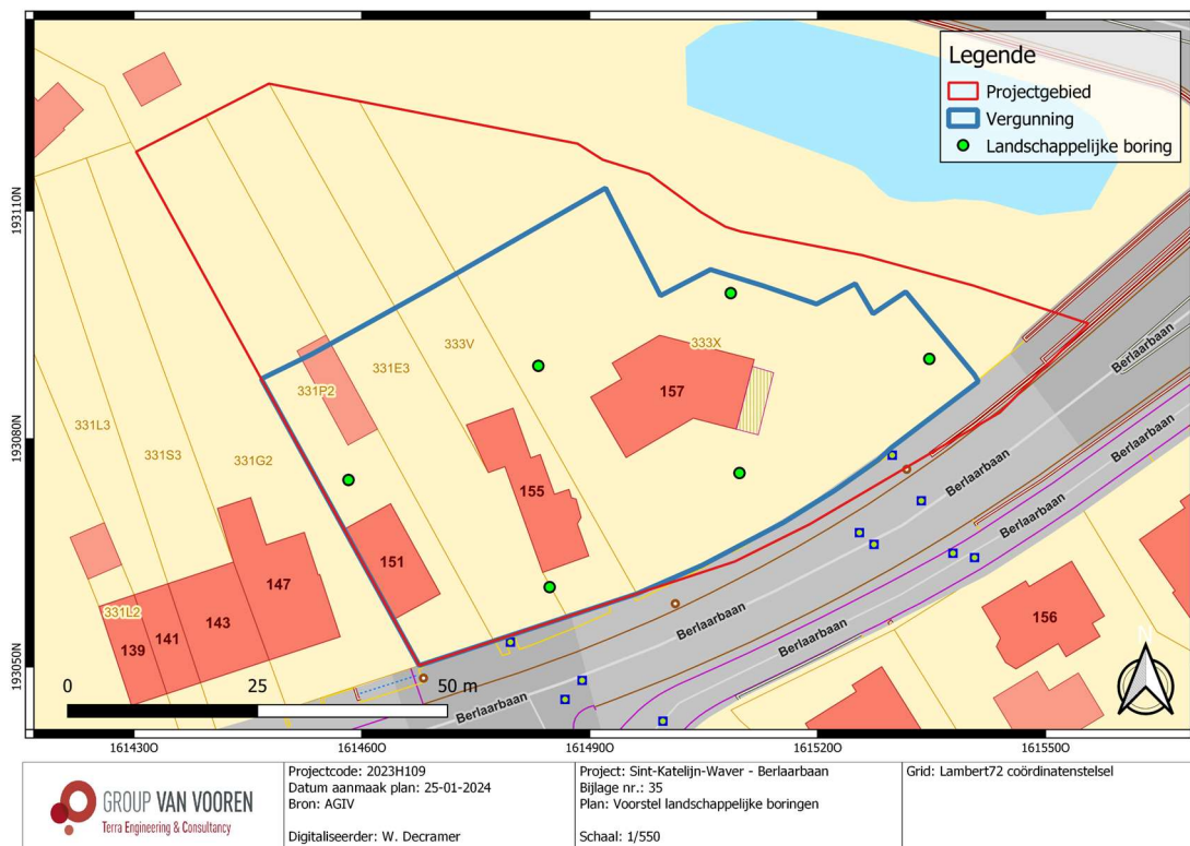
Fig. 2.7: Voorstel boorpuntenplan.
