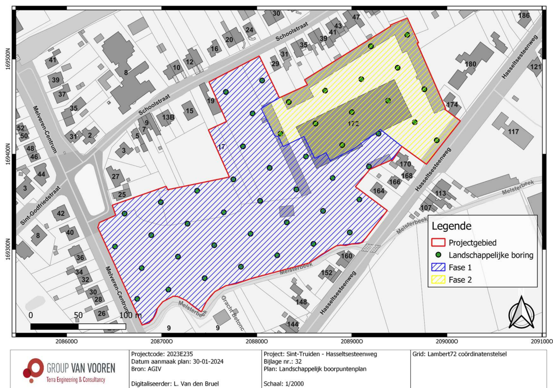
Fig. 2.7: Voorstel boorpuntenplan op het kadaster.
