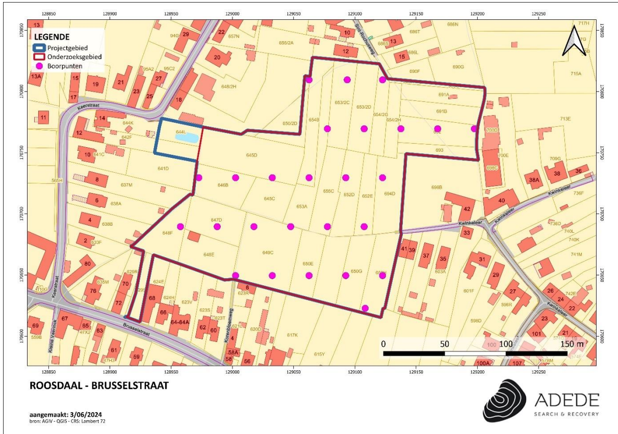
Figuur 2. Boorplan
