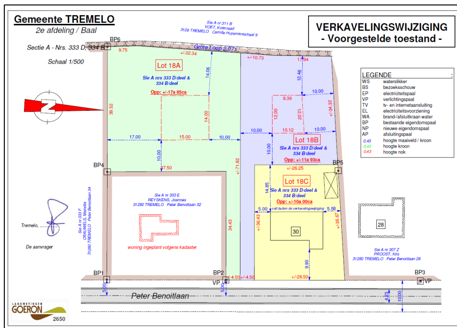
Figuur 8: Voorgestelde toestand (Goeron 2017)
