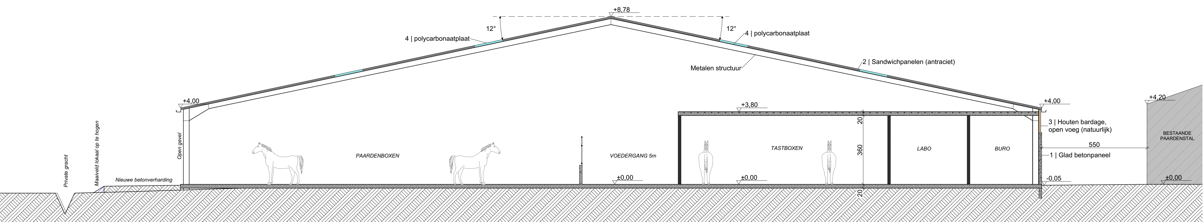
SNEDE A-A NIEUWE TOESTAND - 1:100
