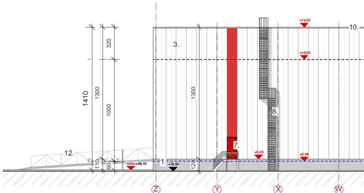
Afb. 3b: Detail met doorsnede die geldig is voor alle hallen. Links een laadkade. Rechts doorsnede van een hal. (Bron: d&d Architects, aanmaakschaal 1.200).
