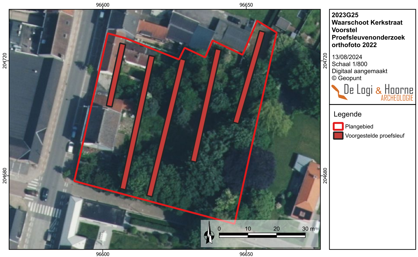
Figuur 33: Indicatief proefsleuvenplan op een recente orthofoto (© Geopunt)
