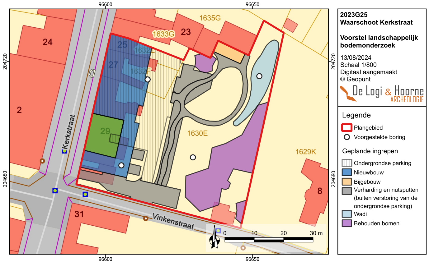
Figuur 30: Indicatief plan voor het landschappelijk bodemonderzoek met aanduiding van de geplande ingrepen (© Geopunt)
