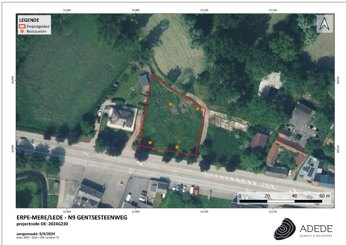
Figuur 4. Boorplan 3
