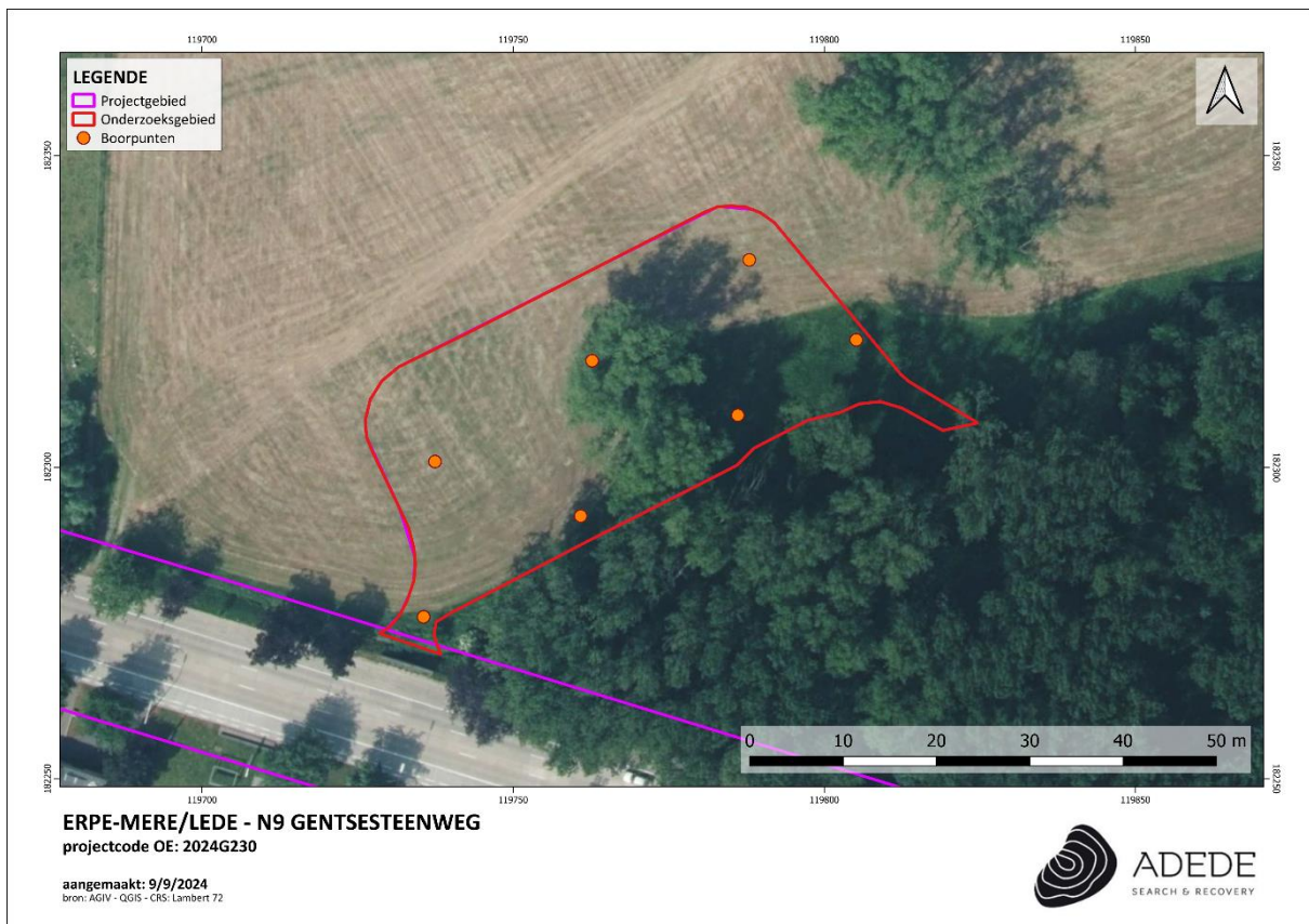
Figuur 2. Boorplan 1
