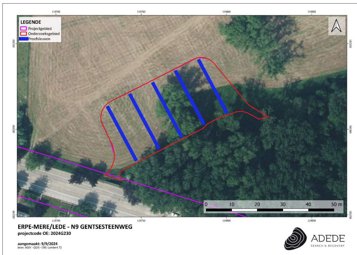
Figuur 6. Proefsleuvenplan 1
