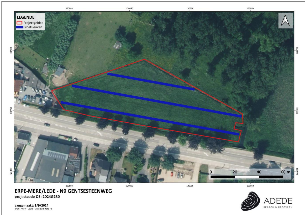
Figuur 7. Proefsleuvenplan 2
