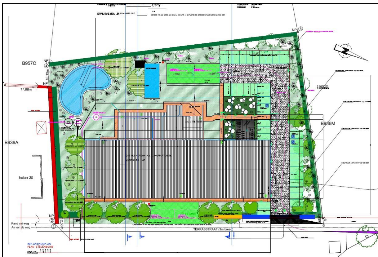
Afb. 4: Inplantingsplan (Bron: initiatiefnemer, digitaal plan, 09/12/2024, aanmaatschaal 1:100, 2024A56)
