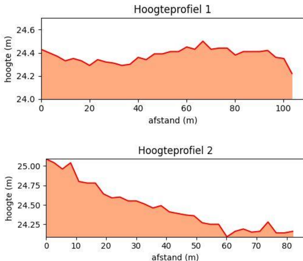
Afb. 9: Hoogteprofiel van het onderzoeksgebied (QGIS/Geopunt, digitaal plan, dd. 05/01/2024, 2024A56).
