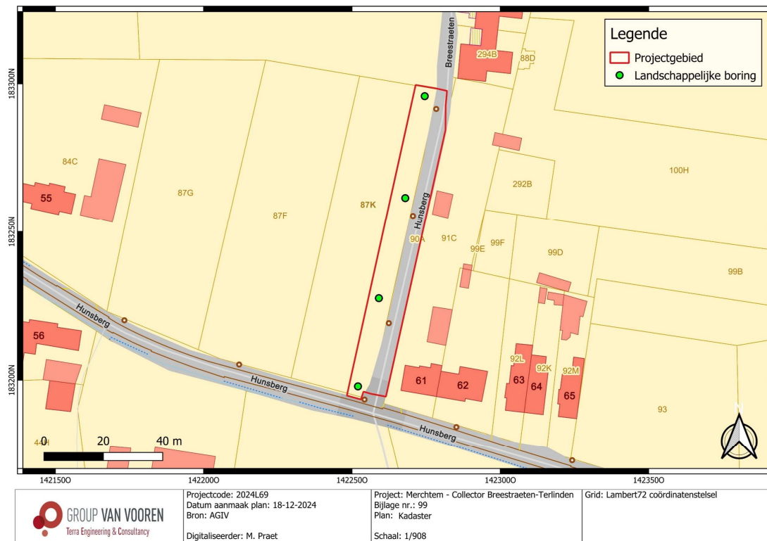
Fig. 2.15: Voorstel boorpuntenplan op het kadasterplan (werkzone Breestraeten-Hunsberg) (© AGIV).
