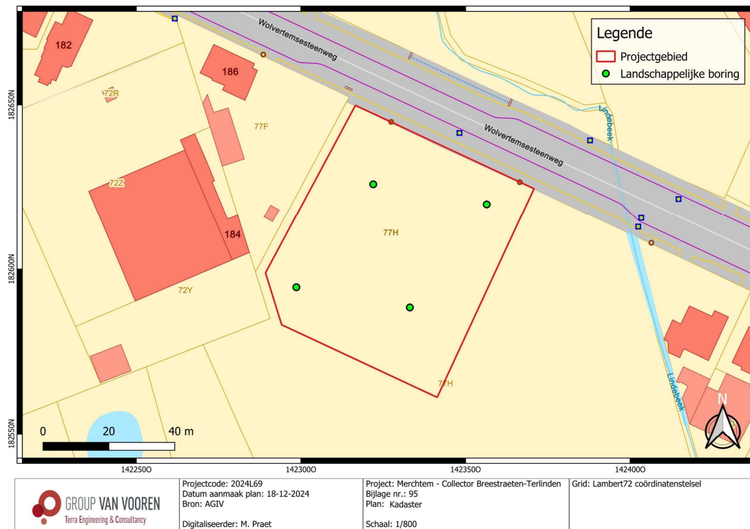
Fig. 2.13: Voorstel boorpuntenplan op het kadasterplan (terrein voor grondverbetering) (© AGIV).
