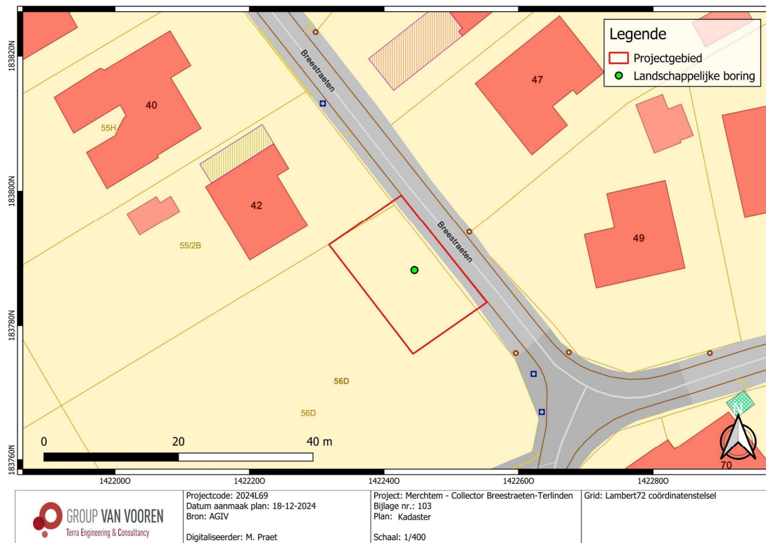
Fig. 2.17: Voorstel boorpuntenplan op het kadasterplan (PS01) (@ AGIV).
