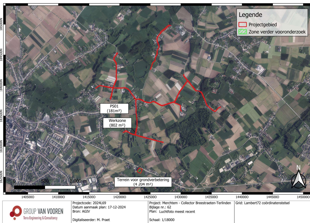
Fig. 2.4: Zone advies vervolgonderzoek geprojecteerd op de meest recente luchtfoto (2023) (overzicht) (© AGIV).
