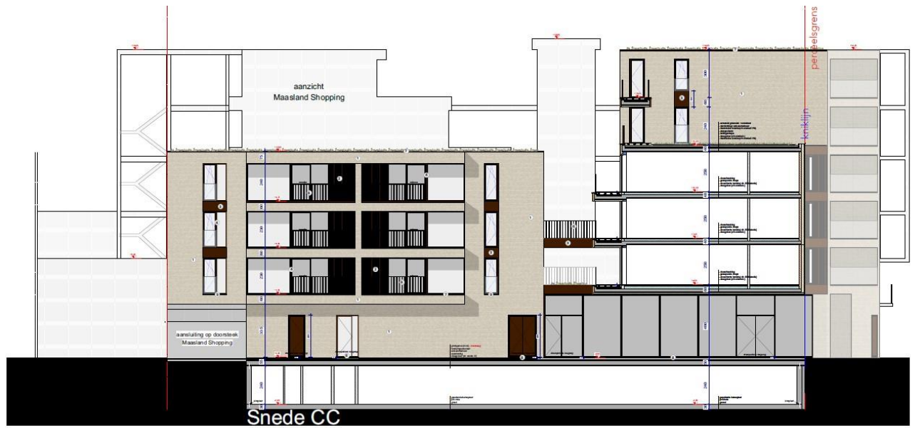
Figuur 5: Snede (Opdrachtgever, 2025)
