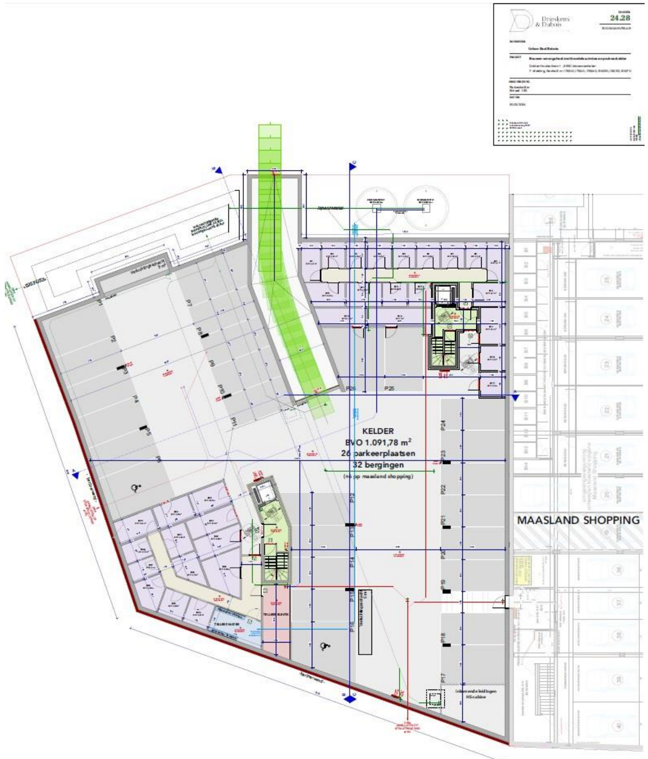
Figuur 3: Kelderplan (Opdrachtgever, 2025)
