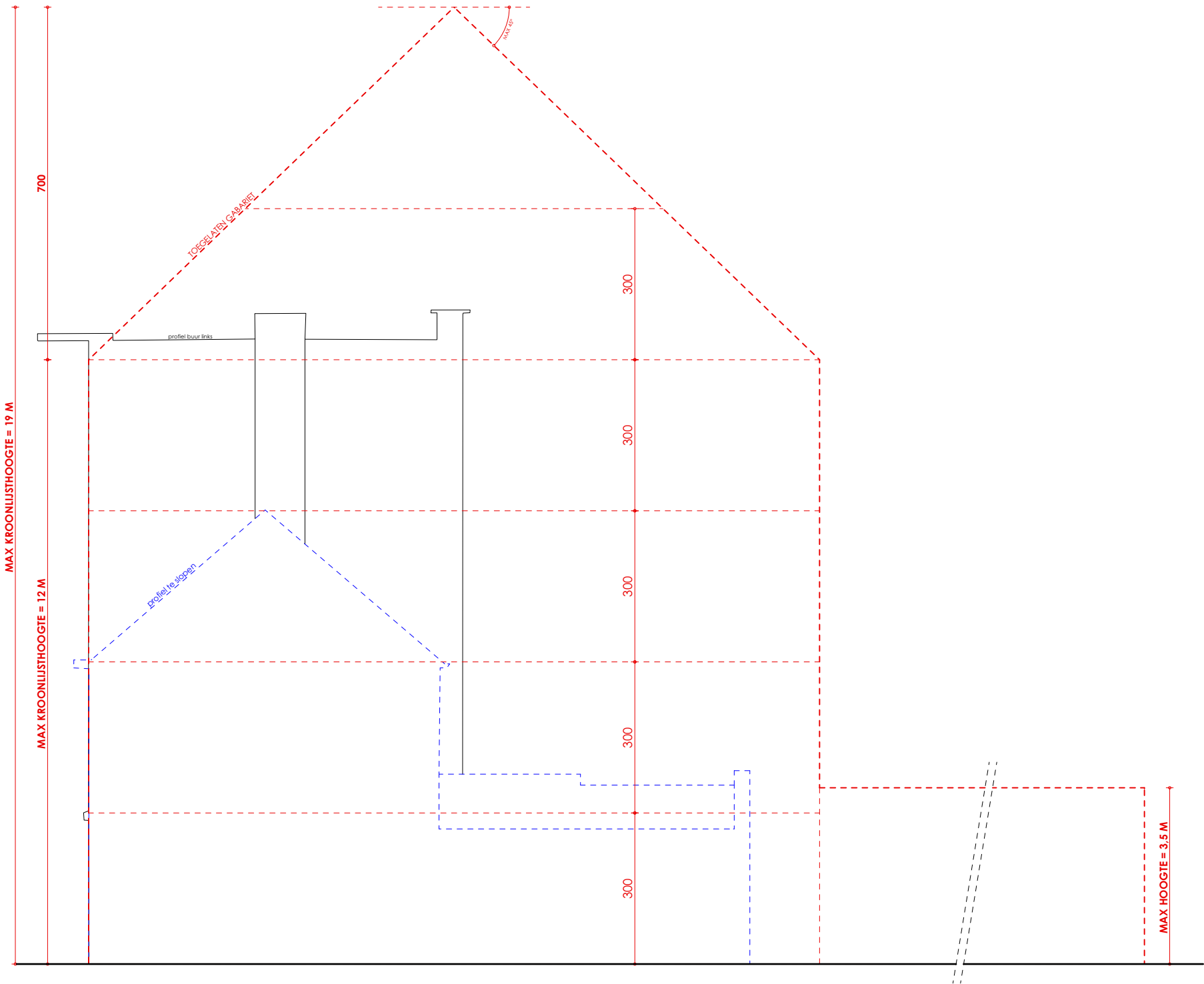
GABARIET BUUR LINKS schaal 1:50
