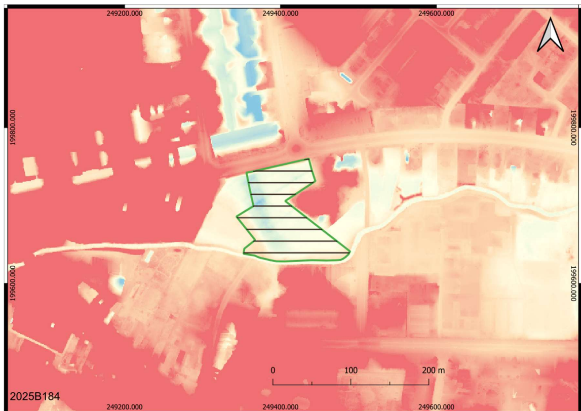
Afbeelding 2: Proefsleuvenplan op de luchtfoto en het DHM.
