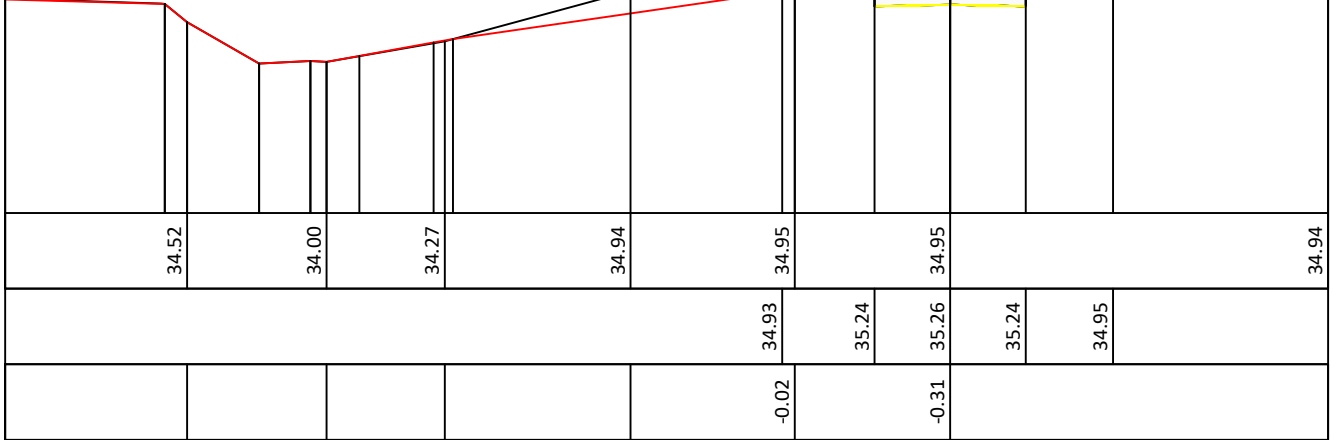
Profiel 8 Vergelijkingsvlak: 32.00 Hoogteschaal: 1
