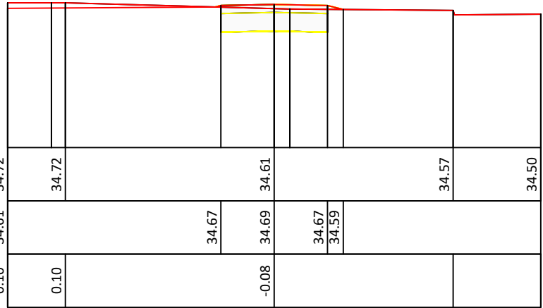
Profiel 2 Vergelijkingsvlak: 32.00 Hoogteschaal: 1
