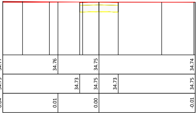
Profiel 3 Vergelijkingsvlak: 32.00 Hoogteschaal: 1
