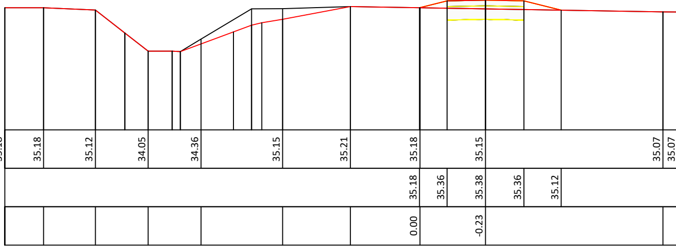
Profiel 9 Vergelijkingsvlak: 32.00 Hoogteschaal: 1
