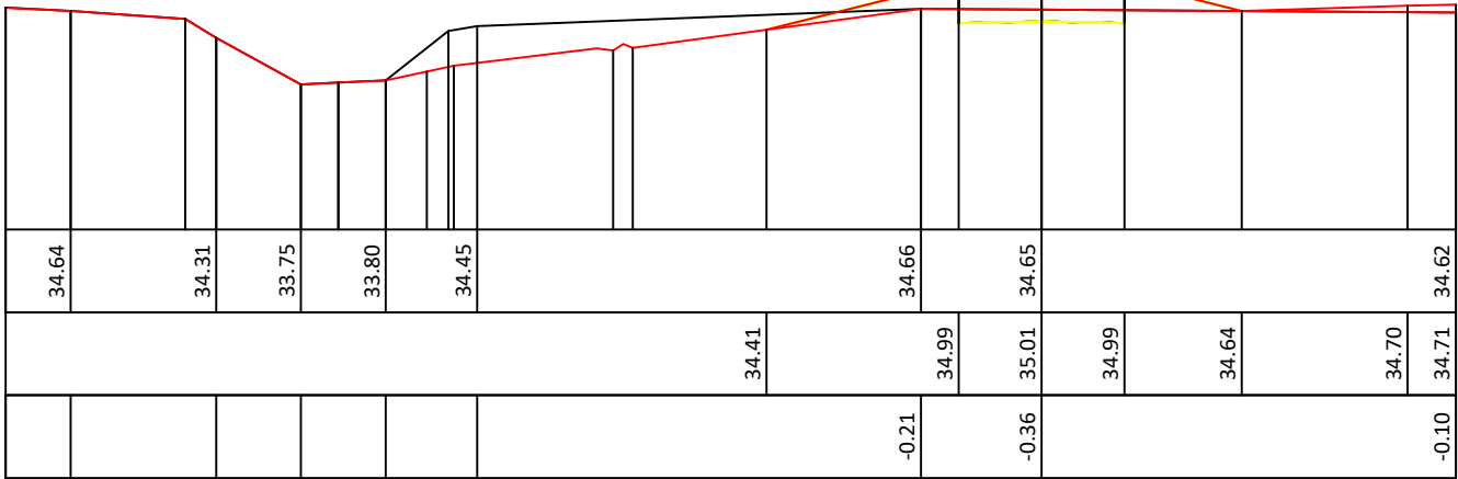
Profiel 6 Vergelijkingsvlak: 32.00 Hoogteschaal: 1
