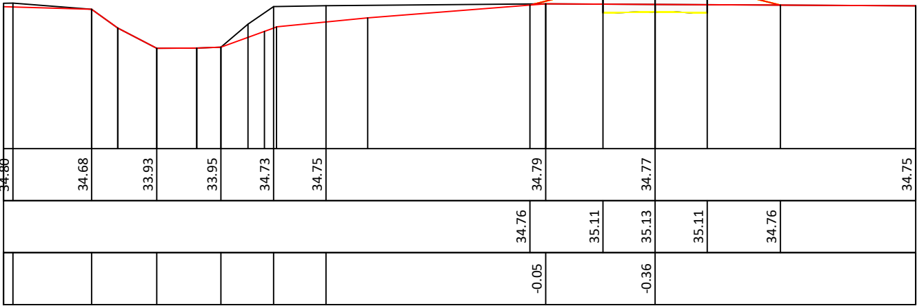
Profiel 7 Vergelijkingsvlak: 32.00 Hoogteschaal: 1
