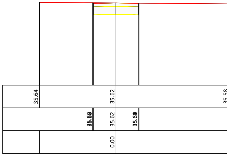
Profiel 11 Vergelijkingsvlak: 32.00 Hoogteschaal: 1
